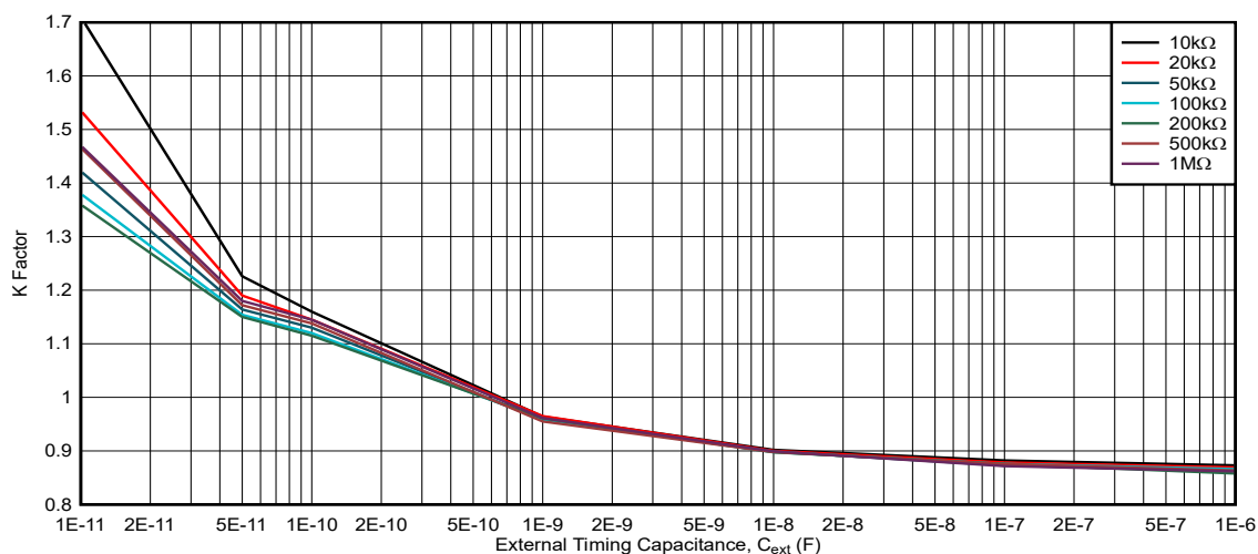
图 5-15. K 系数, V_{CC} = 5.5V , R_{ext} = 10k\Omega 至 1M\Omega
