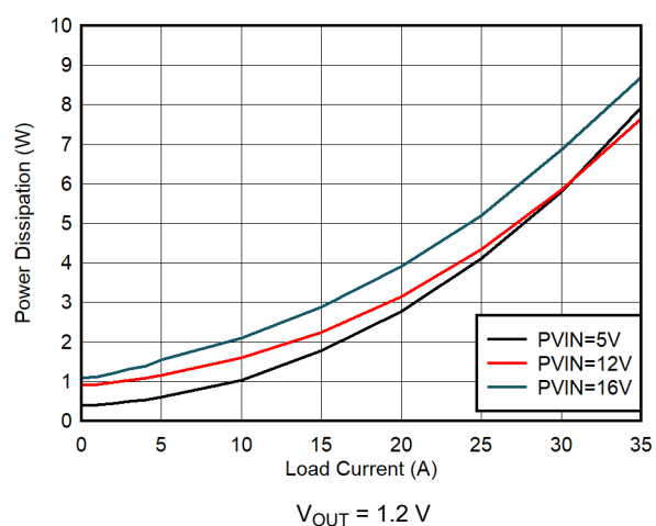
图 9-4. Power Dissipation
