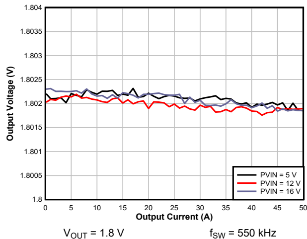
图 8-19. Load Regulation
