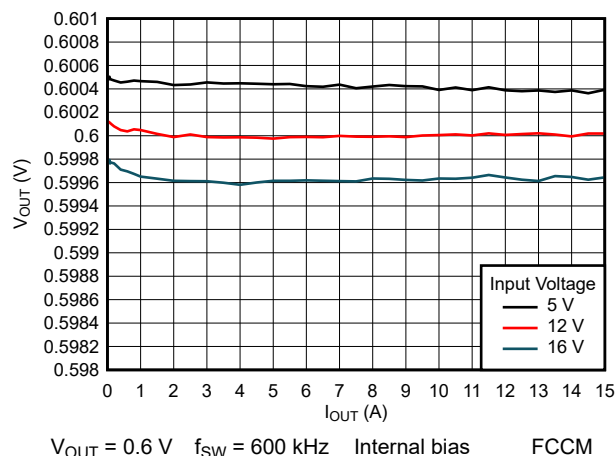
图 8-11. Load Regulation
