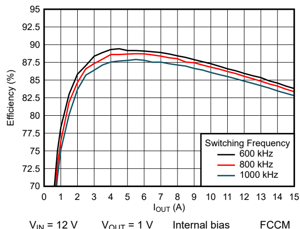
图 8-10. Efficiency
