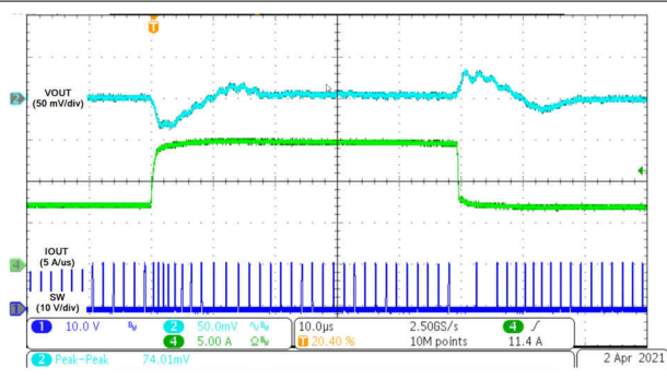
图 8-37. Transient Response, V_{PP} = 74\text{ mV}
