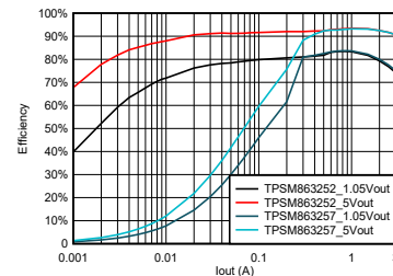
TPSM86325x 在 V_{IN} = 12V 时的效率
