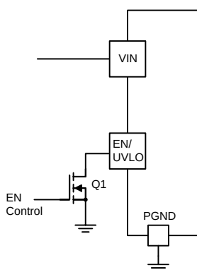
图 15. Enable Control
