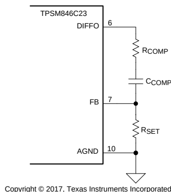
图 15. R SET Resistor
