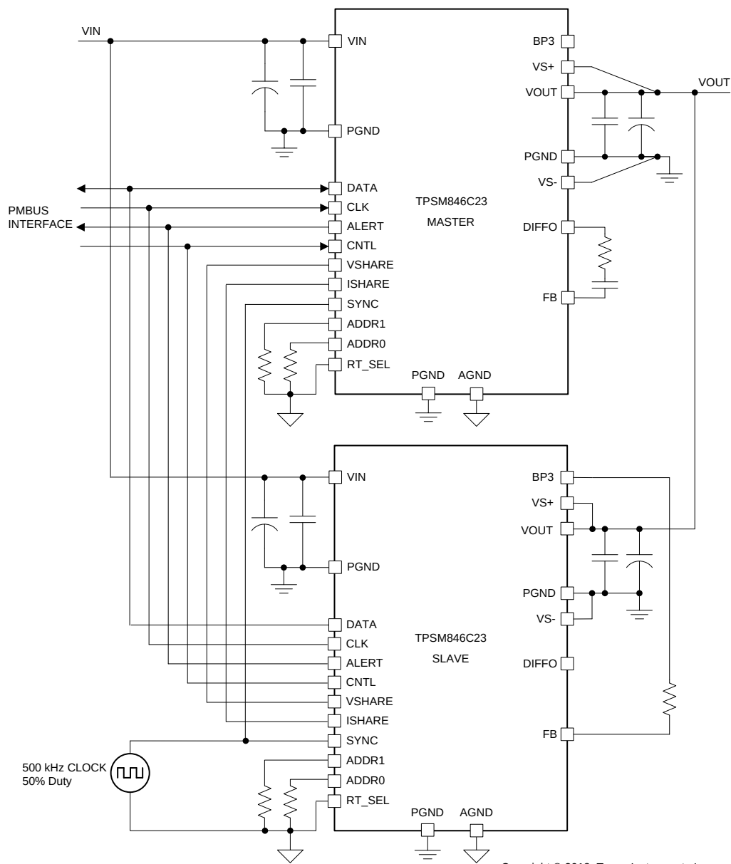
图 18. TPSM846C23 Parallel
