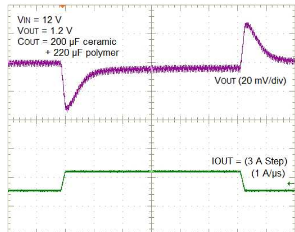
瞬态响应
