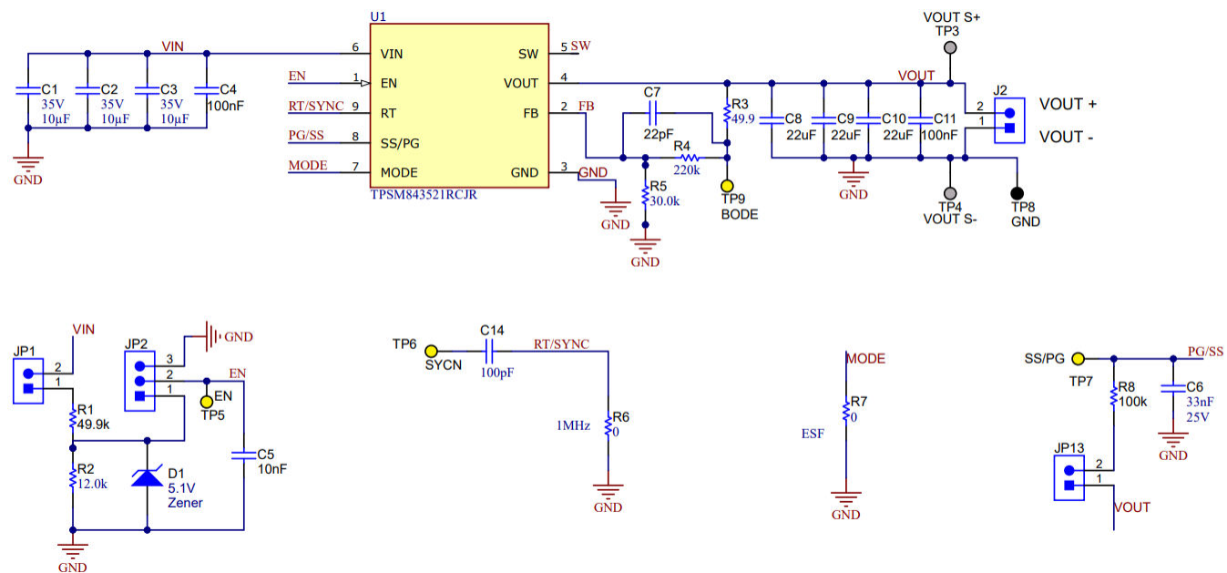
图 7-1. TPSM84538 5V 输出、5A 参考设计
