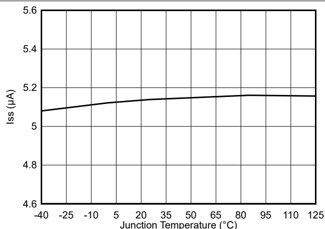
图 5-10. 软启动充电电流与结温间的关系
