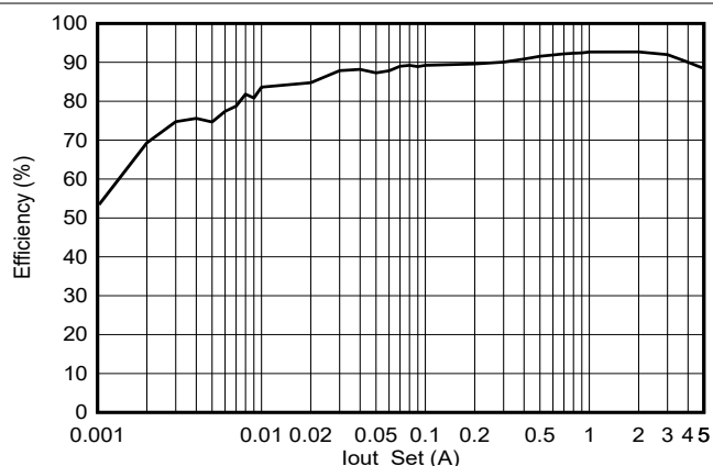
图 7-2. 效率 (PFM)
