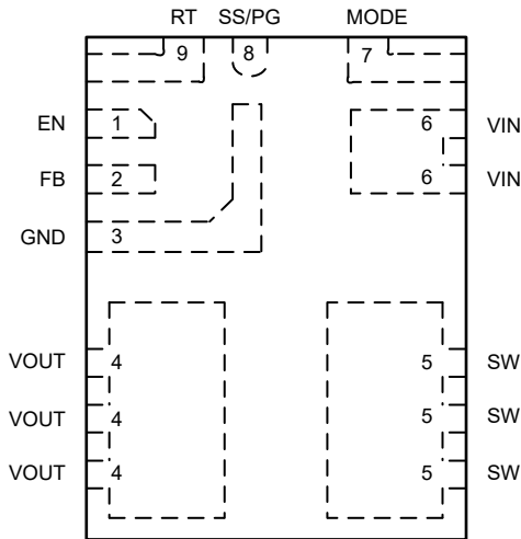
图 4-1.9 引脚 RCJ QFN-FCMOD , 3.3mm × 4.5mm 封装 ( 俯视图 )
