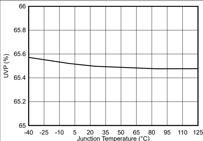
图 5-9. UVP 阈值与结温间的关系
