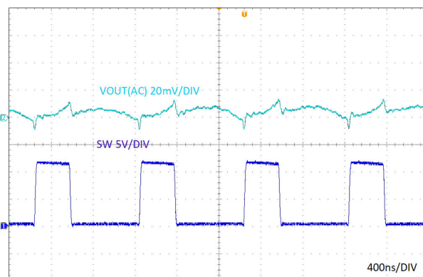
图 7-5. 稳态, I_{OUT} = 5A
