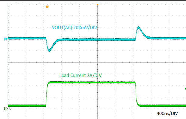
图 7-6. 负载瞬态响应, 0.5A 至 4.5A , 压摆率 = 0.8A/\mu S
