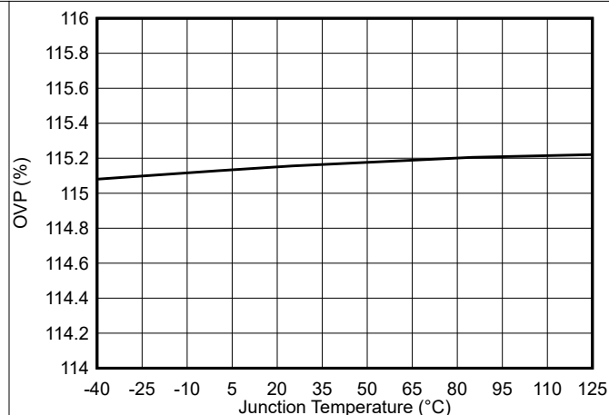
图 5-8. OVP 阈值与结温间的关系
