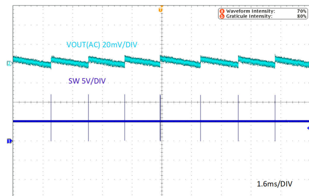
图 7-4. 稳态, I_{OUT} = 0A
