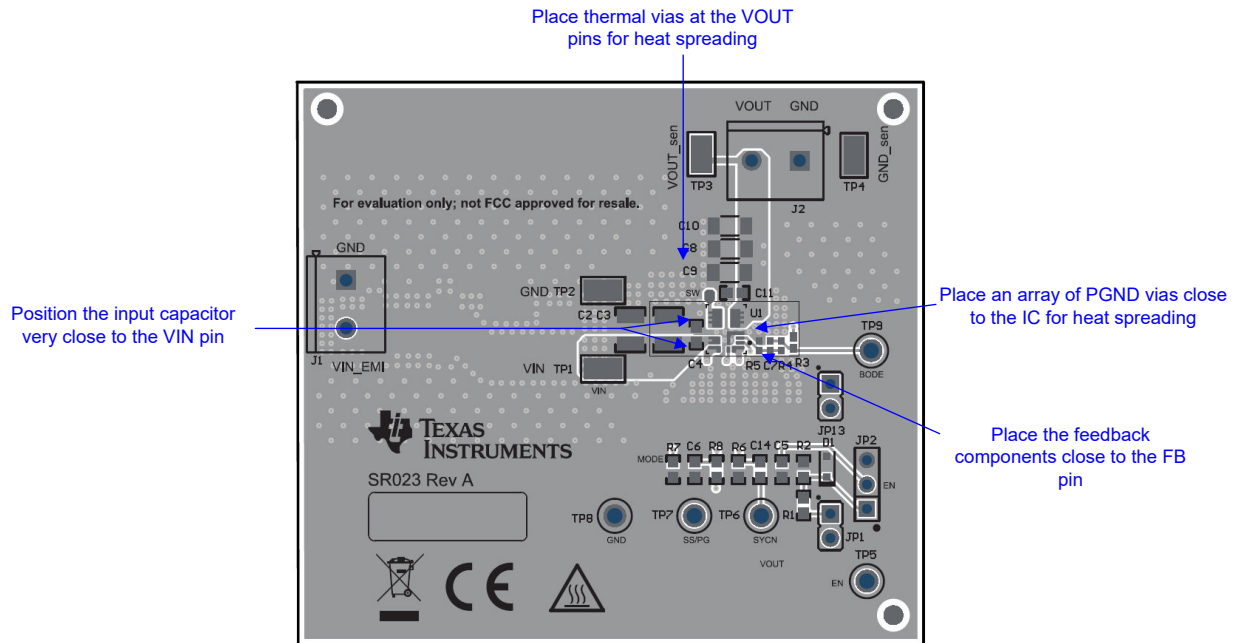
图 7-9. TPSM84538 顶层布局示例
