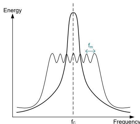
图 6-8. 能量与频率间的关系
