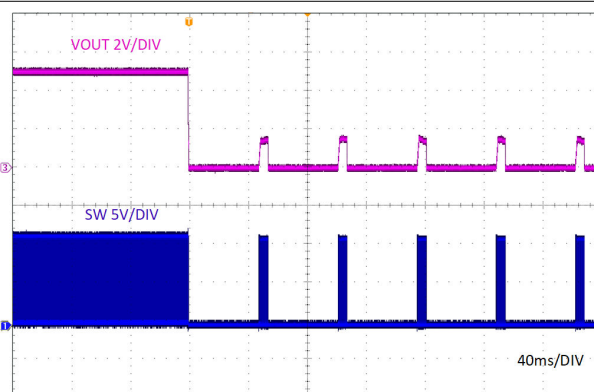
图 7-7. V_{OUT} 硬短路保护
