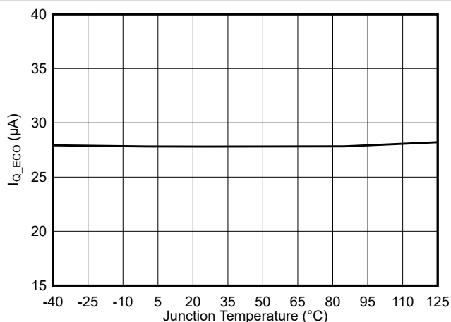
图 5-1. TPSM84538 静态电流 (PFM) 与结温间的关系
