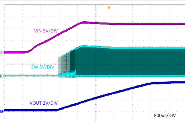
图 7-3. 相对于 V_{IN} 、 I_{OUT} = 5A 的启动
