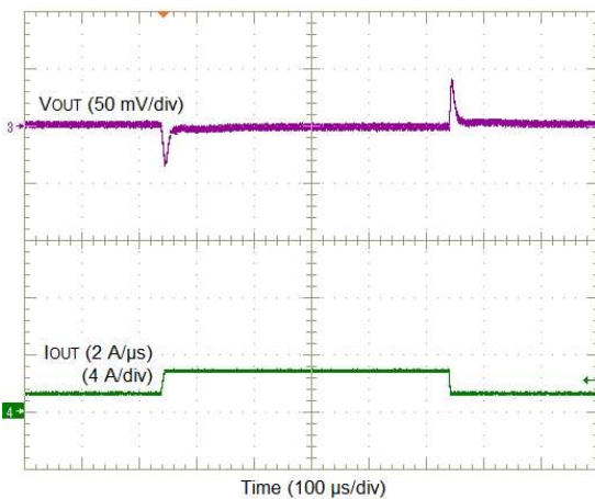
图 16. V_{OUT} = 1\text{ V} , 2-A Load Step
