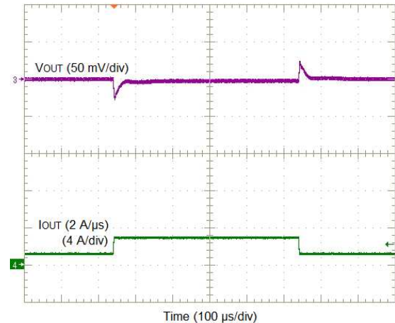
图 15. V_{OUT} = 0.8\text{ V} , 2-A Load Step
