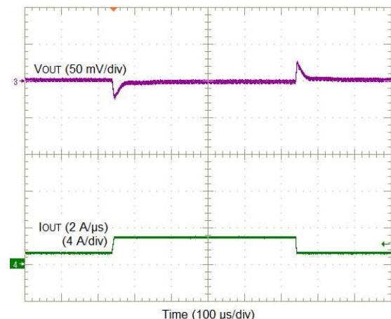
图 17. V_{OUT} = 1\text{ V} , 2-A Load Step
