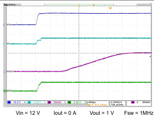
图 8-9. EN 启动 - 测量 BP5
