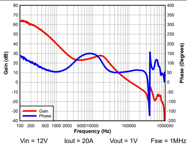
图 8-7. 波特图
