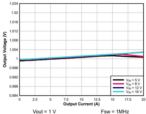
图 8-5. 负载调整率
