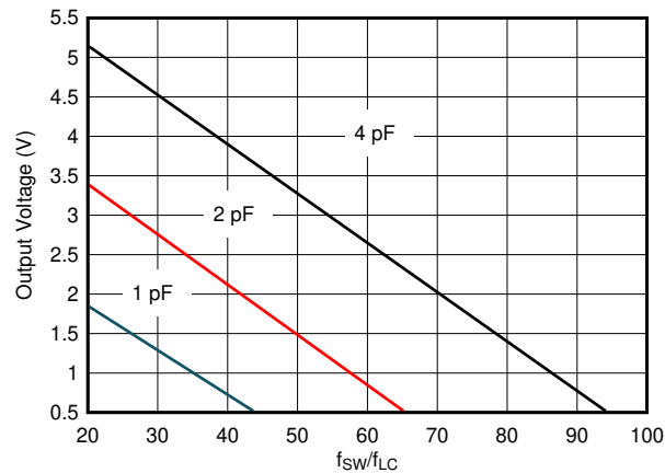
图 8-3. 推荐的斜坡设置
