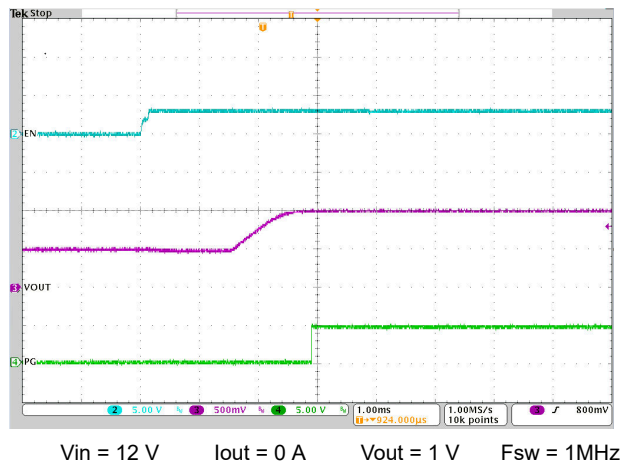
图 8-12. EN 启动 - 0.5V 预偏置
