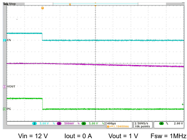
图 8-10. EN 关断
