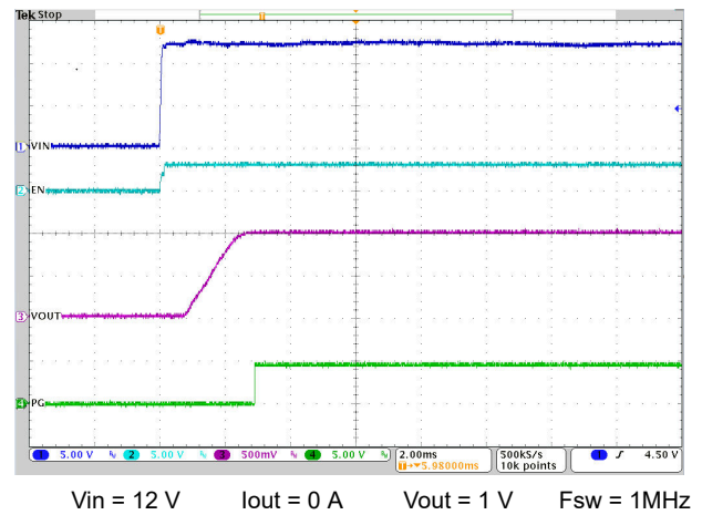
图 8-13. VIN 启动
