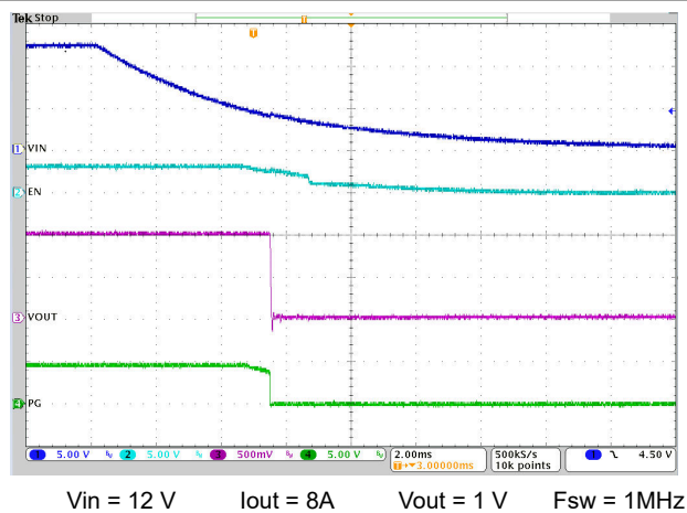
图 8-14. VIN 关断
