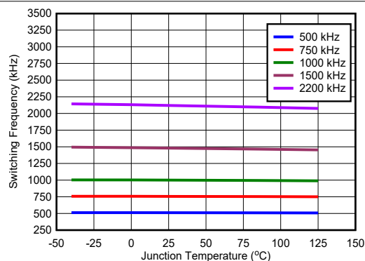
图 6-16. 开关频率与温度间的关系
