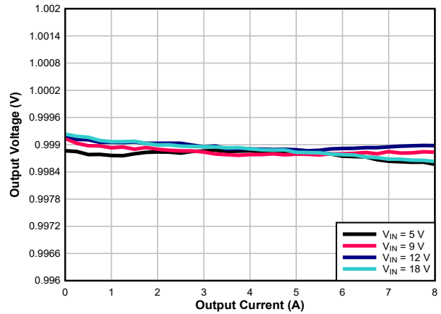
图 7-5. Load Regulation
