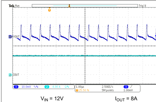
图 7-16. Output Ripple – 8A Load
