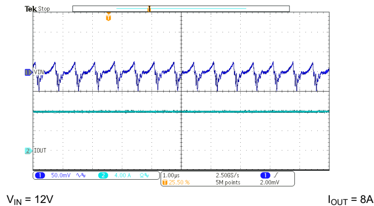
图 7-18. Input Ripple – 8A Load
