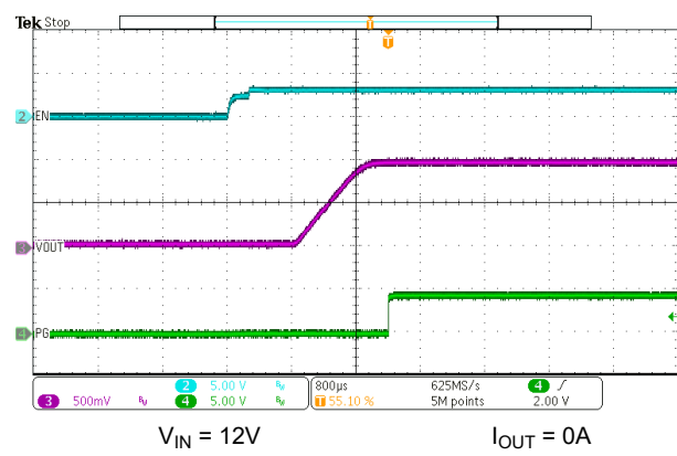
图 7-9. EN Start-Up – No Load
