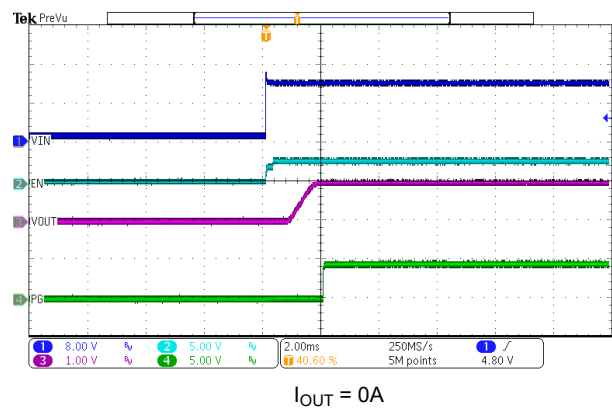
图 7-13. VIN Start-Up
