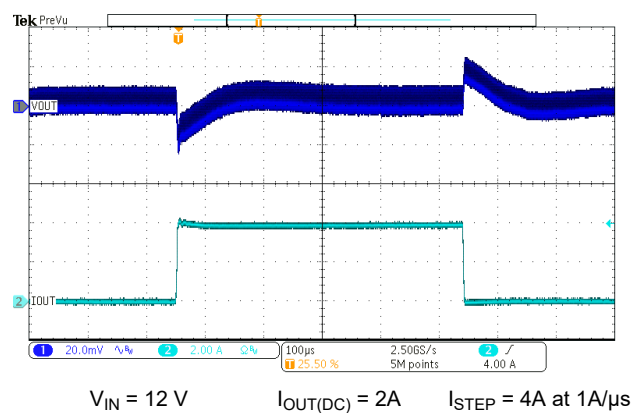
图 7-8. Load Transient
