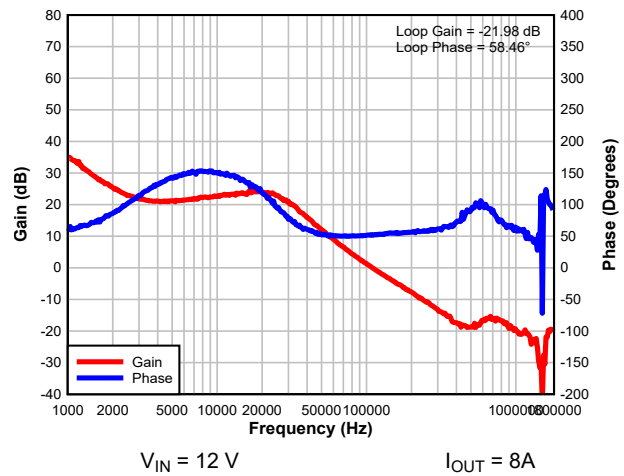
图 7-7. Bode Plot
