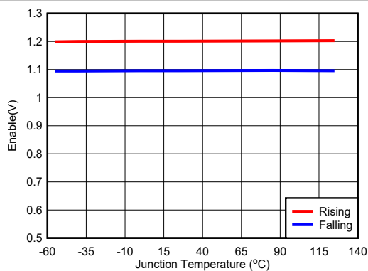
图 5-5. Enable Voltage
