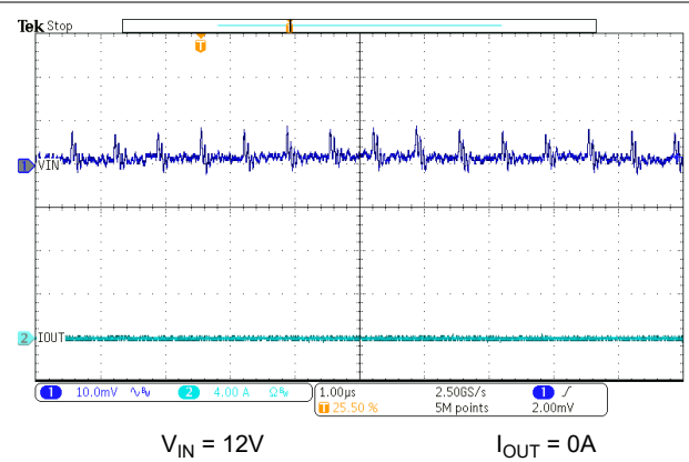
图 7-17. Input Ripple – No Load
