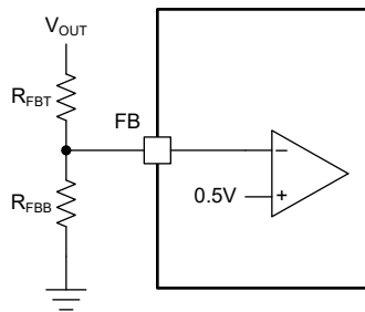
图 6-3. FB Resistor Divider
