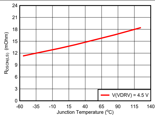
图 5-2. Low-Side FET RdsON
