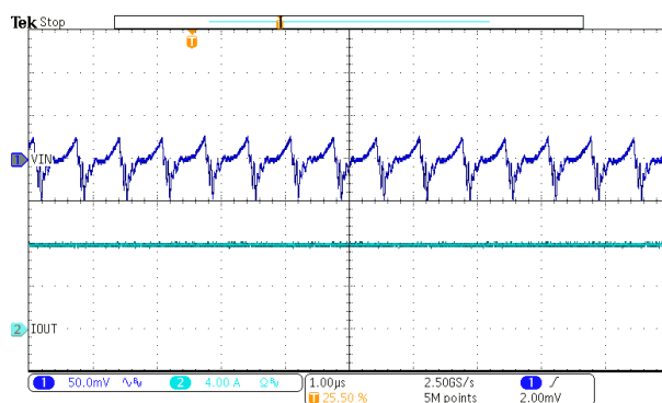
图 7-16. Output Ripple – 8-A Load
