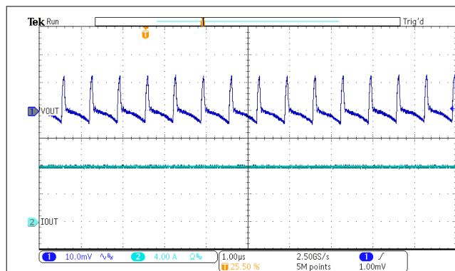
图 7-16. Output Ripple – 8-A Load
