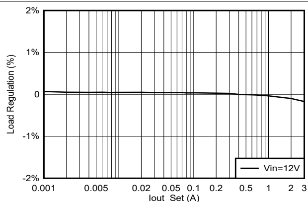
图 7-3. 负载调节 (ECO)
