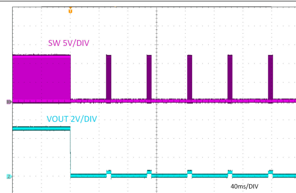
图 7-7. V_{OUT} 硬短路保护
