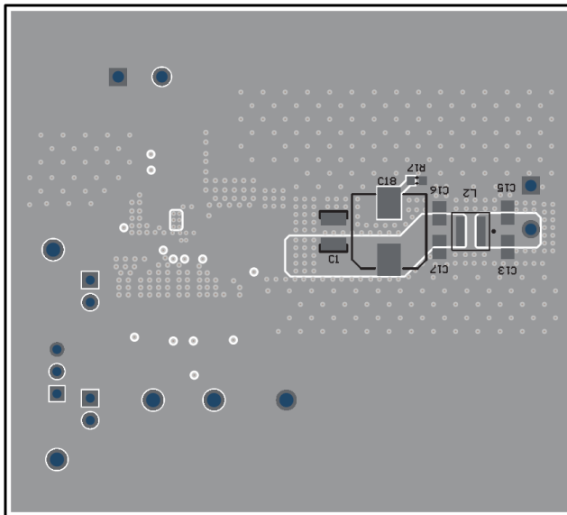
图 7-10. TPSM843321 底层布局示例
