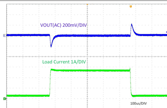
图 7-6. 负载瞬态响应, 0.3A 至 2.7A , 压摆率 = 0.8A/\mu S
