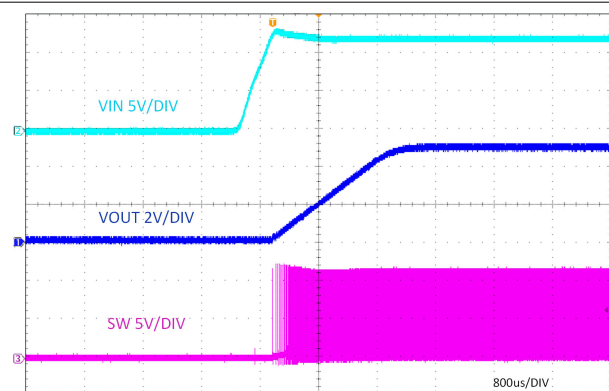
图 7-4. 相对于 V_{IN} 、 I_{OUT} = 3A 的启动
