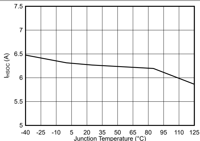
图 5-9. TPSM843321 高侧电流限值与结温间的关系
