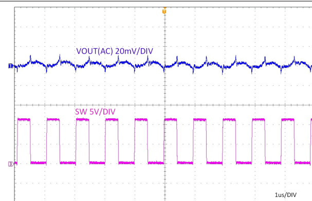
图 7-5. 稳态, I_{OUT} = 3A
