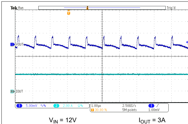
图 7-16. Output Ripple – 3A Load
