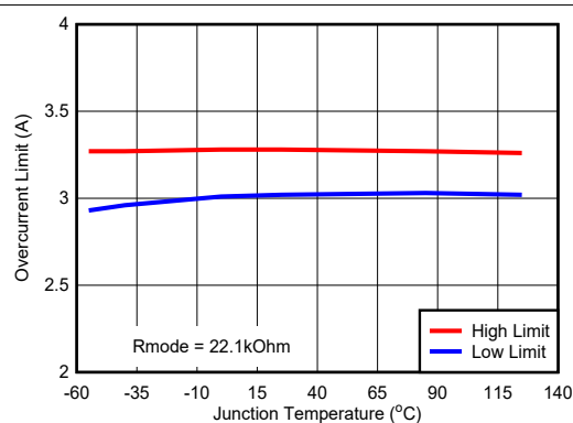
图 5-4. Overcurrent Limit : R = 22.1kOhm
