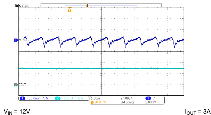
图 7-18. Input Ripple – 3A Load
