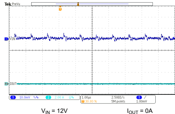
图 7-17. Input Ripple – No Load
