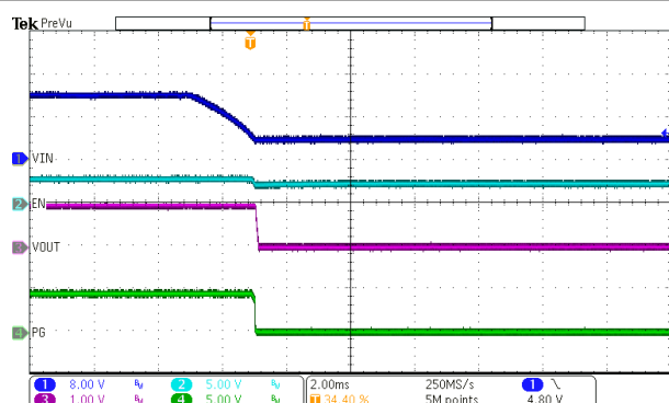
I_{OUT} = 3A 图 7-14. VIN Shutdown
