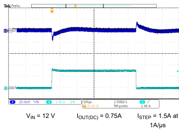
图 7-8. Load Transient
