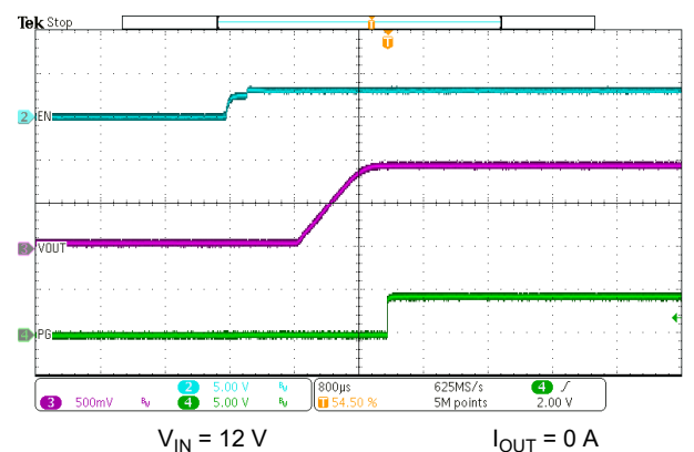
图 7-9. EN Start-Up - No Load
