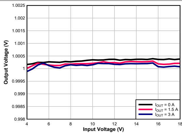
图 7-6. Line Regulation
