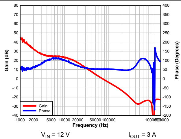
图 7-7. Bode Plot
