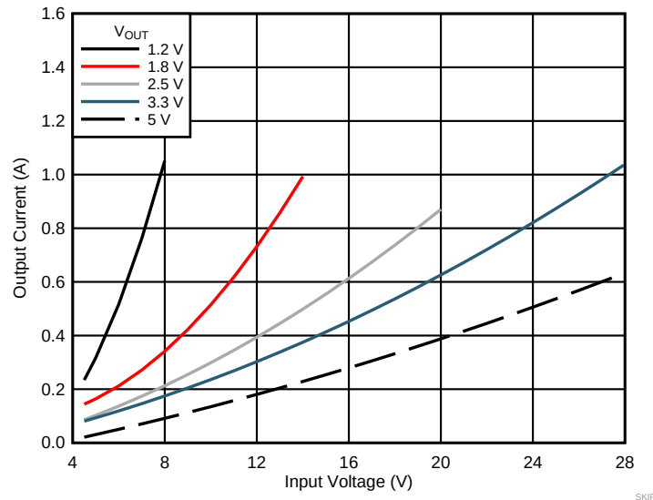
图 26. Pulse-Skipping Threshold
