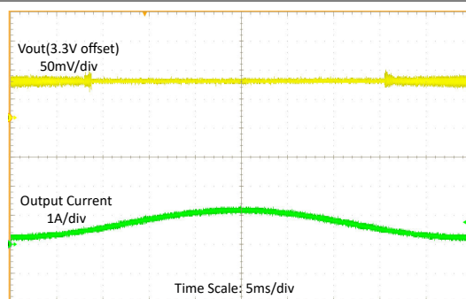
图 8-15. 输入电压为 3.6V 时的负载扫描
