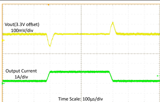
图 8-12. 输入电压为 2.7V 时的负载瞬态
