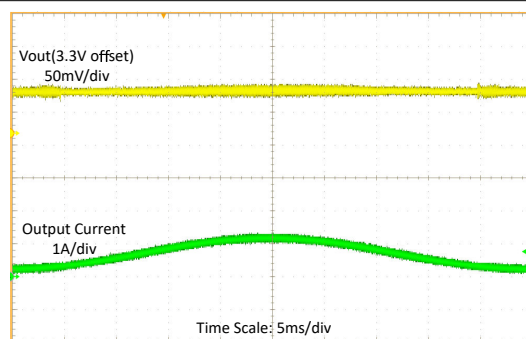
图 8-13. 输入电压为 2.7V 时的负载扫描
