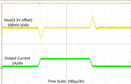
图 8-14. 输入电压为 3.6V 时的负载瞬态
