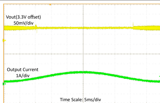
图 8-17. 输入电压为 4.3V 时的负载扫描
