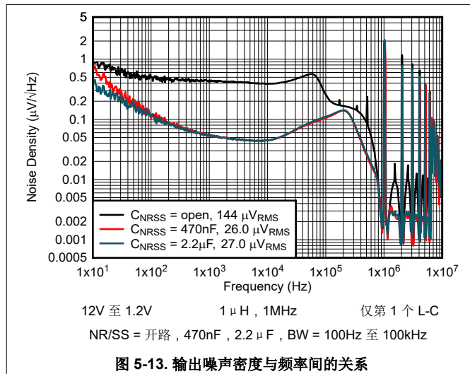
图 5-13. 输出噪声密度与频率间的关系
