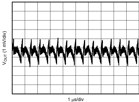
图 5-5. 第 1 个 L-C 滤波器之后的 V_{OUT} 纹波
