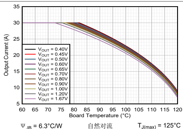
图 9-34. TPSM8287B30xx 安全工作区, V_{IN} = 3.3V
