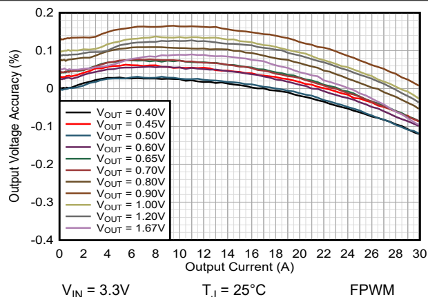
图 9-16. TPSM8287B30xx 负载调整率
