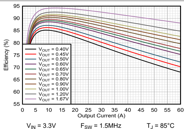
图 9-40. 效率 TPSM8287B30xx FPWM
