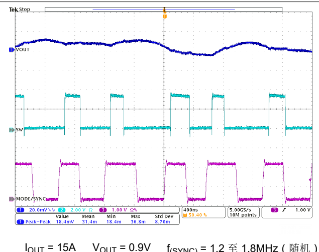
图 9-27. 与随机外部时钟同步
