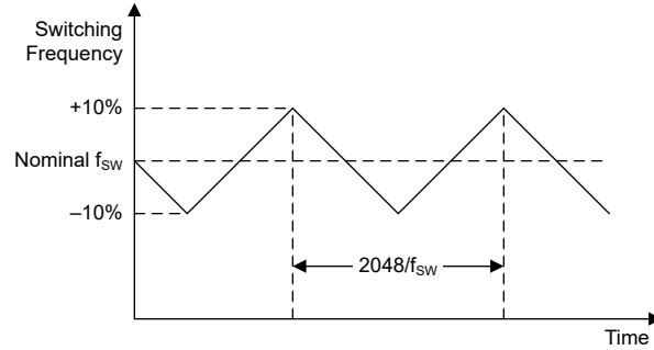
图 7-11. 展频时钟行为
