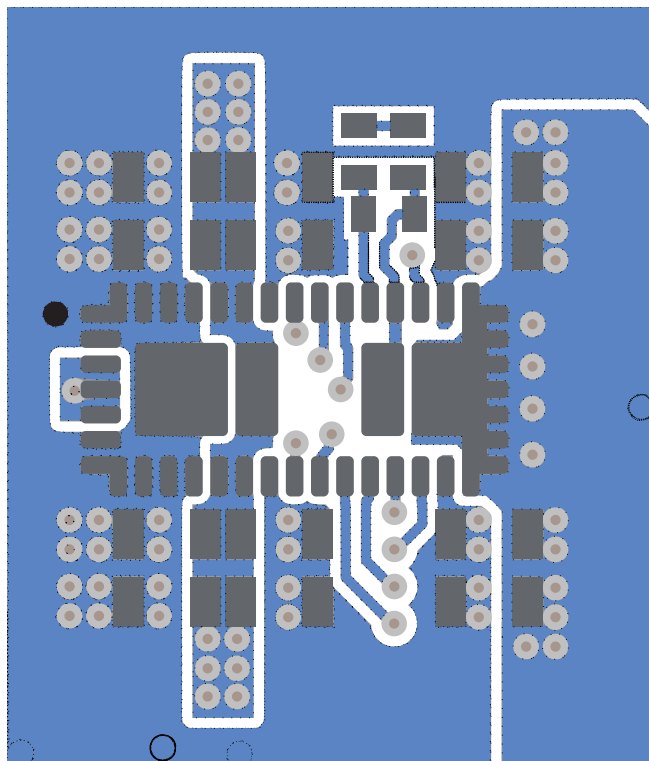
图 9-43. 布局示例
