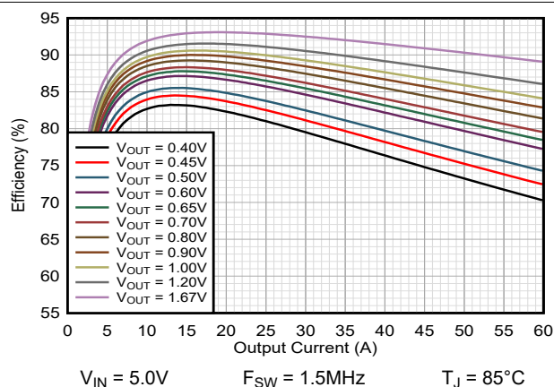
图 9-42. 效率 TPSM8287B30xx FPWM
