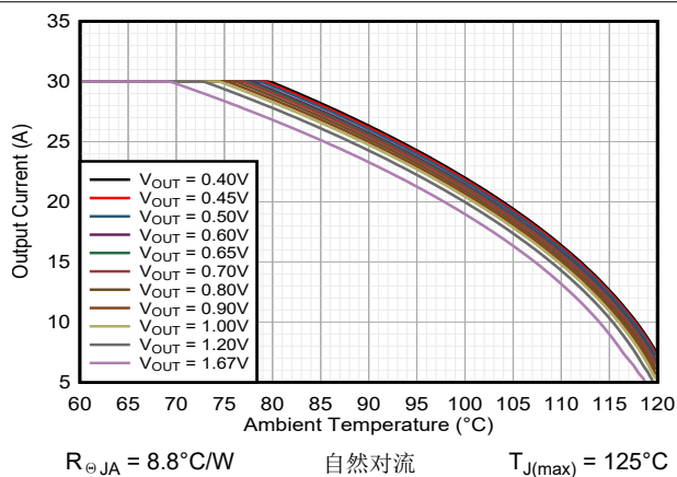
图 9-33. TPSM8287B30xx 安全工作区, V_{IN} = 5.0V
