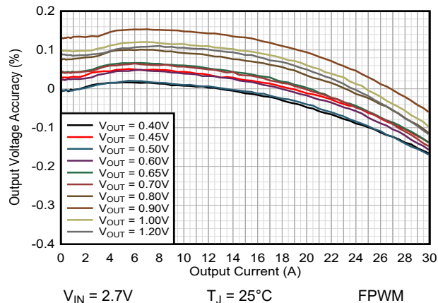
图 9-14. TPSM8287B30xx 负载调整率
