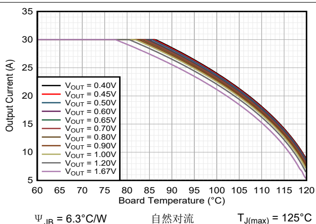
图 9-35. TPSM8287B30xx 安全工作区, V_{IN} = 5.0V
