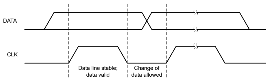
图 7-19. 串行接口上的位传输
