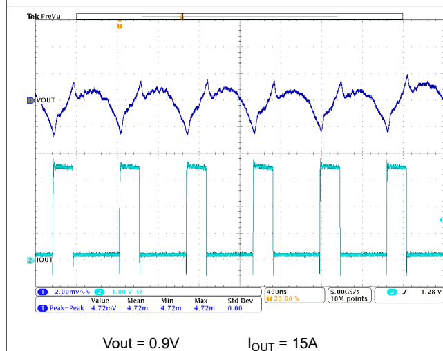
图 9-22. TPSM8287B30xx PWM-CCM 运行
