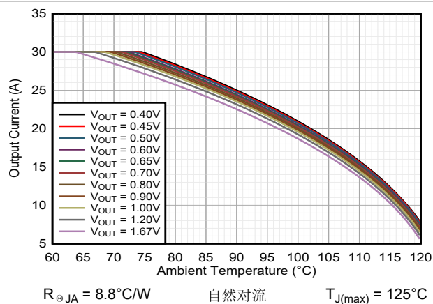
图 9-32. TPSM8287B30xx 安全工作区, V_{IN} = 3.3V
