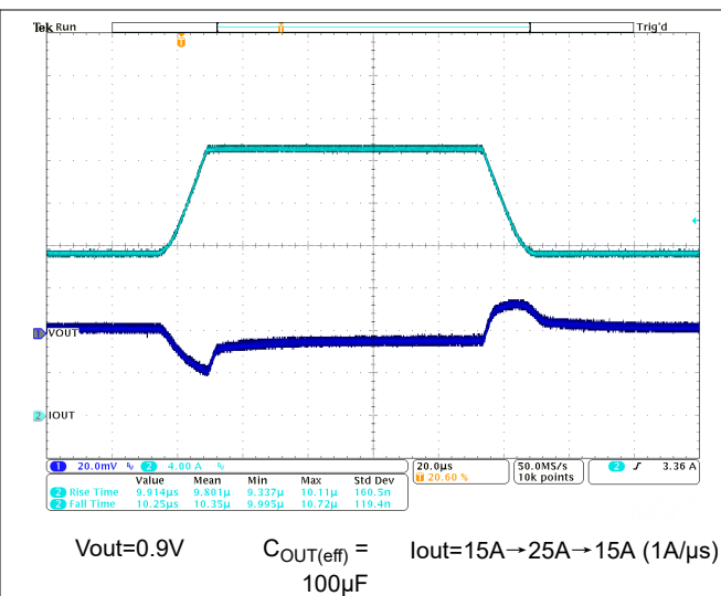
图 9-21. 负载瞬态 TPSM8287B30xx
