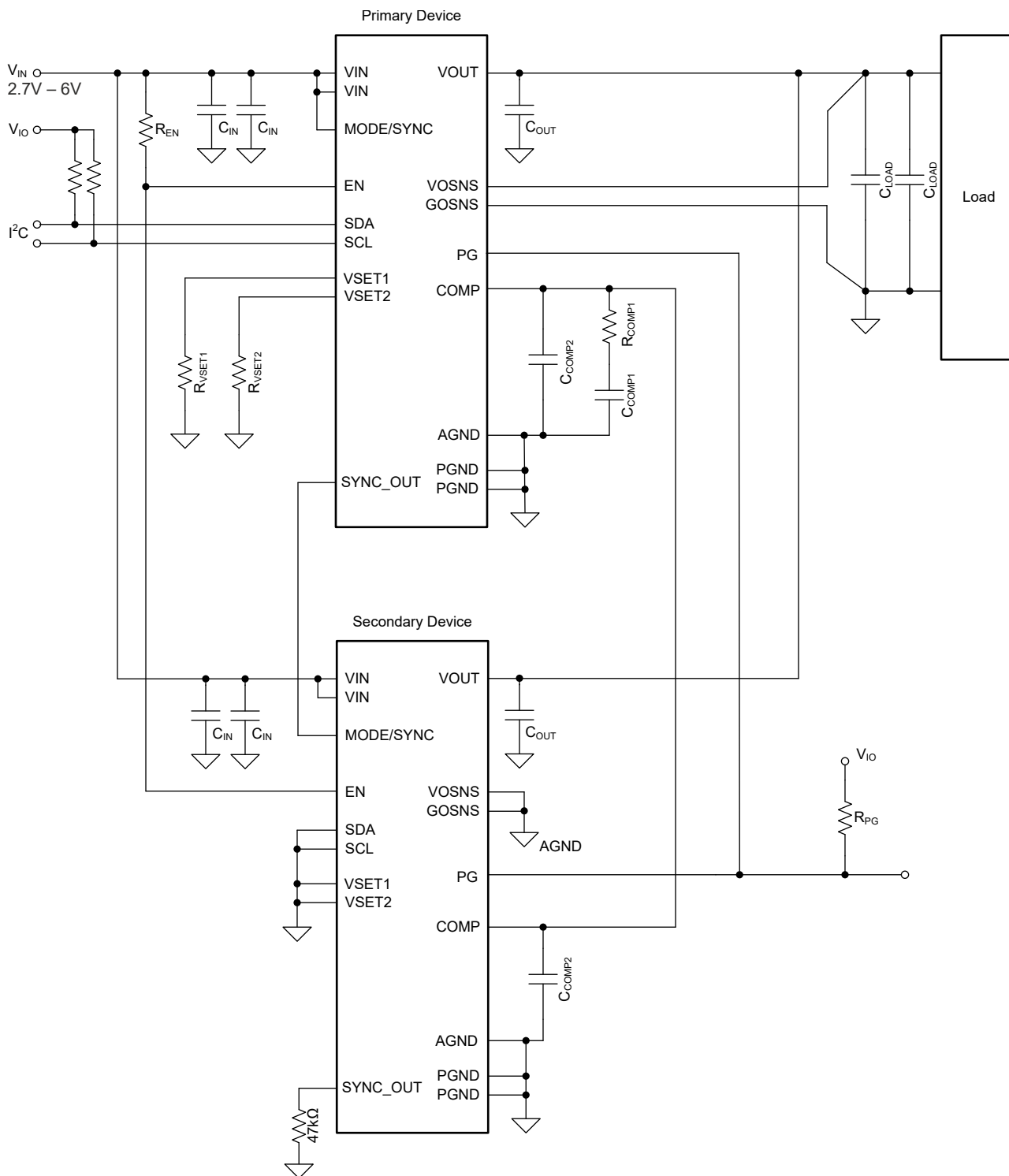
图 7-17. 堆叠配置中的两个 TPSM8287Bxx 器件
