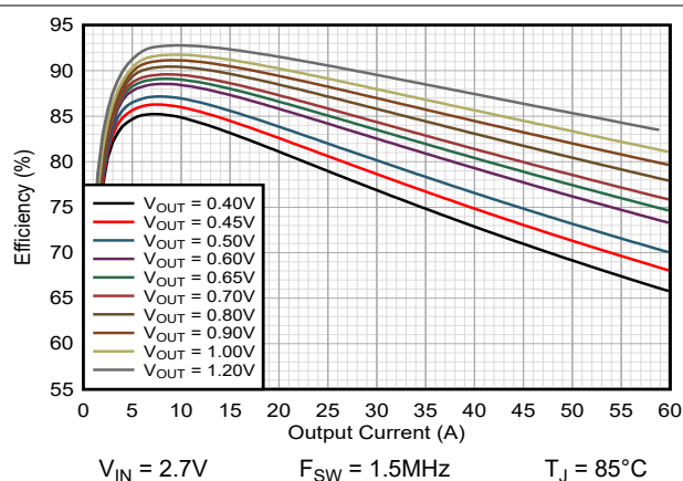
图 9-38. 效率 TPSM8287B30xx FPWM
