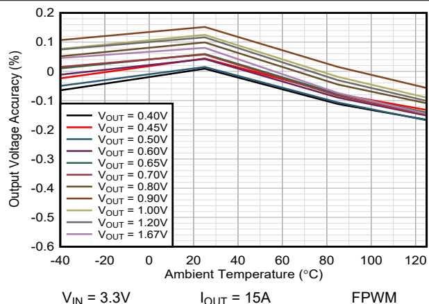
图 9-17. TPSM8287B30xx Vout 精度与温度间的关系
