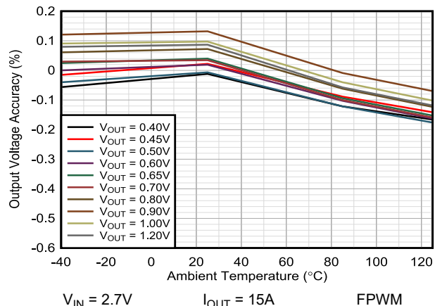
图 9-15. TPSM8287B30xx Vout 精度与温度间的关系
