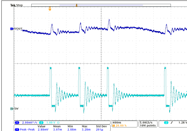
图 9-24. TPSM8287B30xx PFM-DCM 运行
