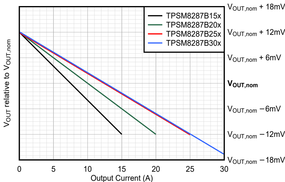
图 7-10. 电压随输出电流的调节
