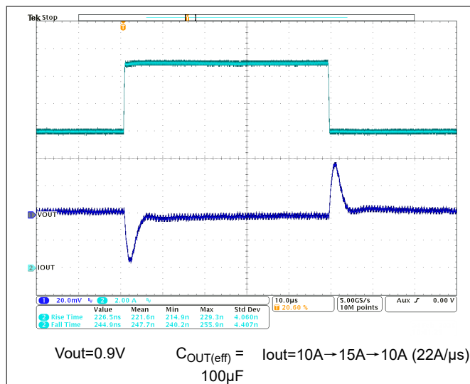
图 9-20. 负载瞬态 TPSM8287B30xx
