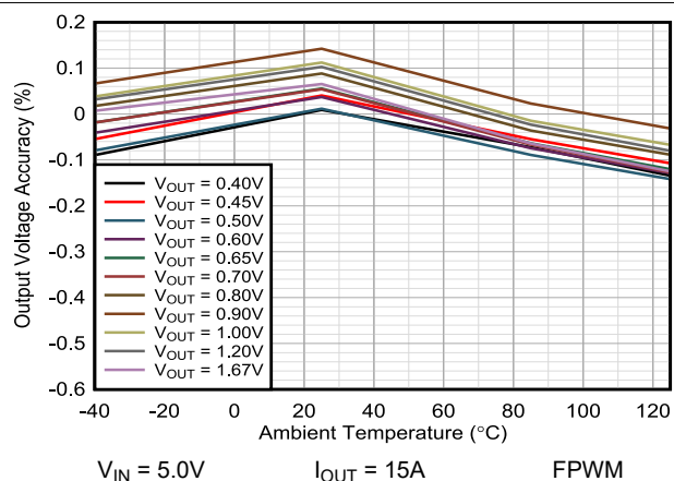
图 9-19. TPSM8287B30xx Vout 精度与温度间的关系
