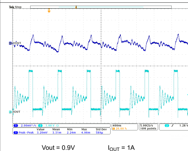
图 9-23. TPSM8287B30xx PWM-DCM 运行
