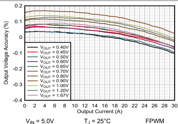
图 9-18. TPSM8287B30xx 负载调整率
