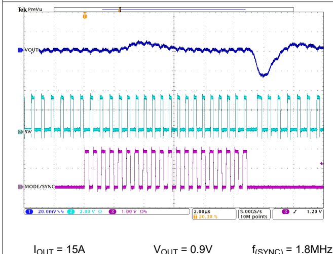
图 9-26. 添加和移除外部时钟
