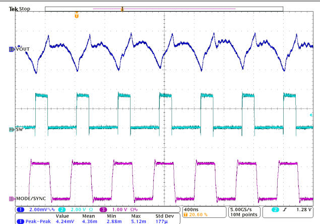
图 9-25. 可与外部时钟保持同步
