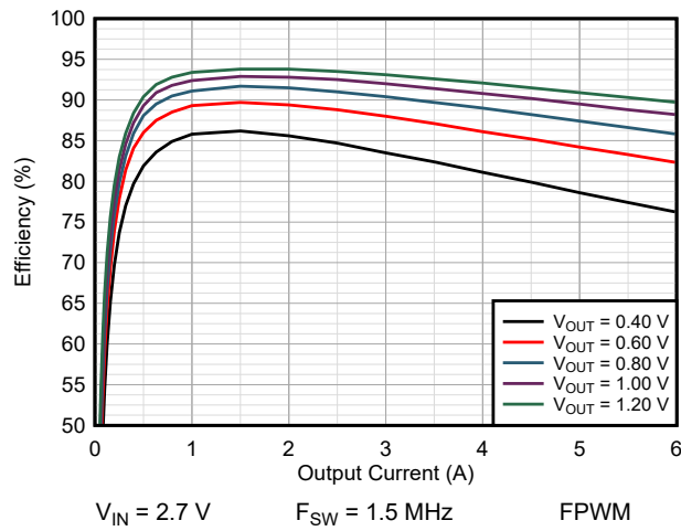
图 9-2. Efficiency TPSM8287A06BAS
