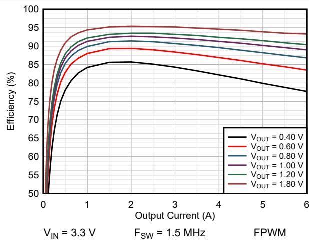
图 9-4. Efficiency TPSM8287A06BAS
