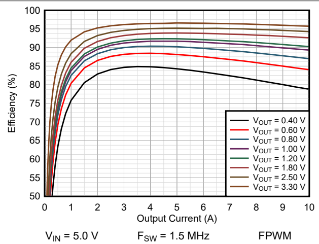
图 9-7. Efficiency TPSM8287A10BAH
