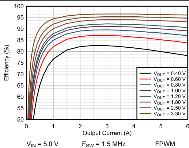
图 9-6. Efficiency TPSM8287A06BAS
