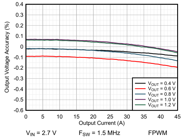
图 9-52. Load Regulation
