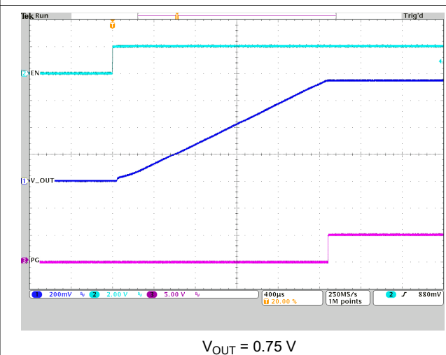
图 9-35. Start-Up Using EN Pin
