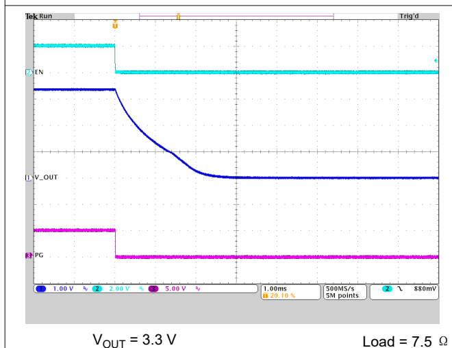
图 9-36. Shutdown Using EN Pin (Discharge Enabled)
