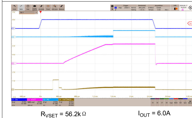
图 9-22. 满载启动
