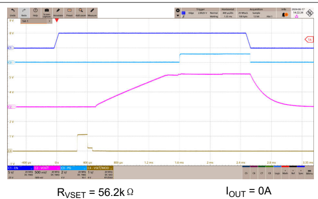
图 9-23. 空载启动
