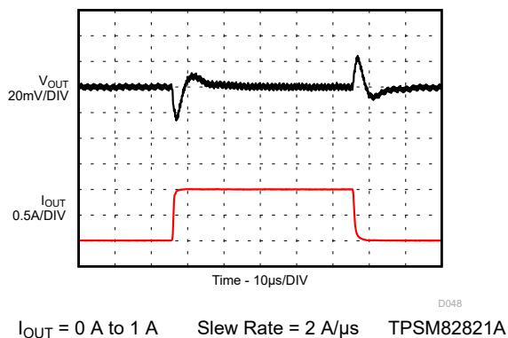
图 9-49. Load Transient
