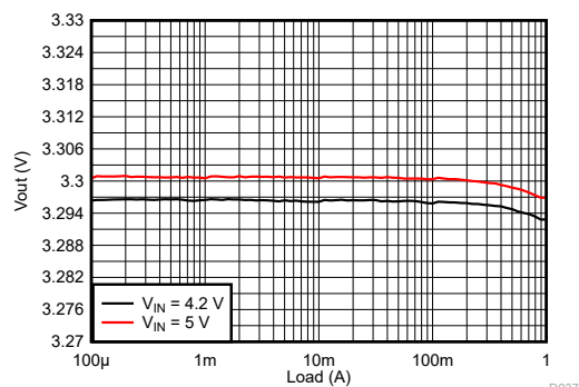
图 9-44. Load Regulation
