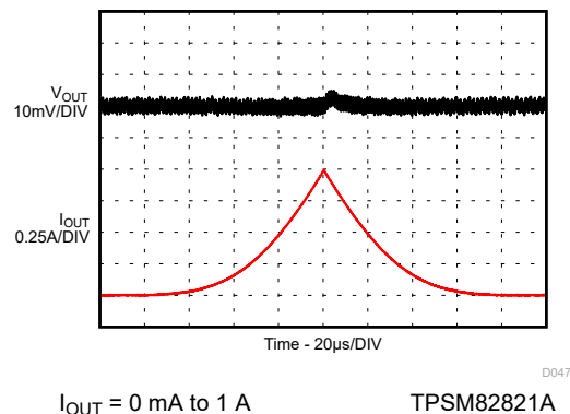
图 9-48. Load Sweep
