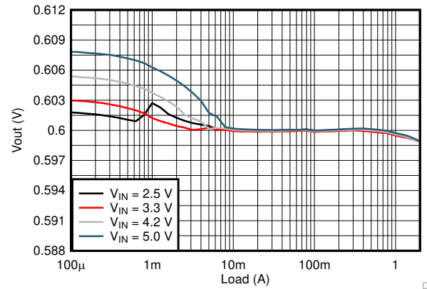
图 9-66. Load Regulation
