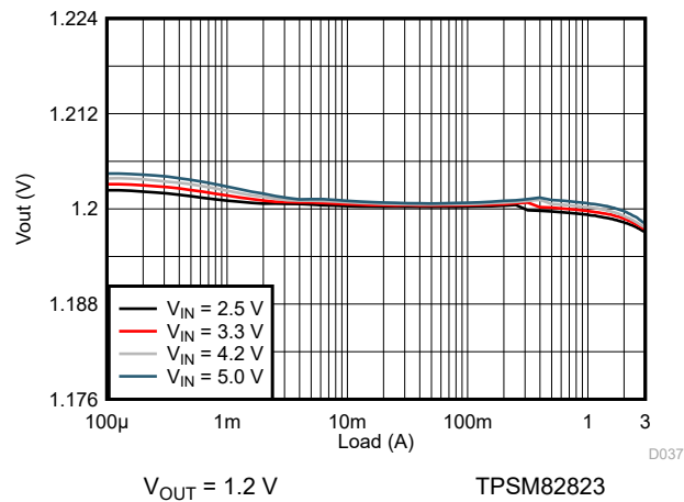
图 9-124. Load Regulation
