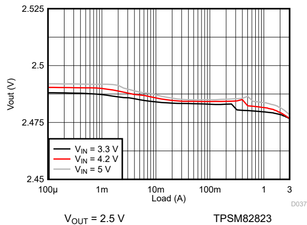
图 9-126. Load Regulation
