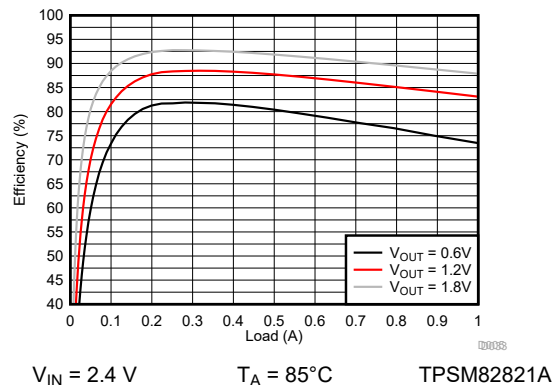
图 9-36. Efficiency
