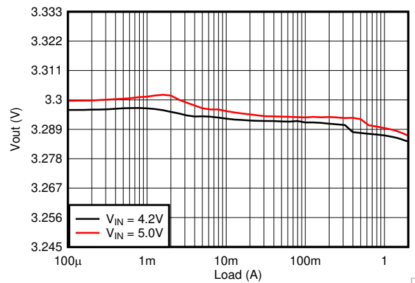
图 9-68. Load Regulation
