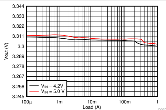
图 9-18. Load Regulation
