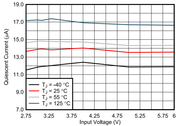
图 6-1. Quiescent Current
