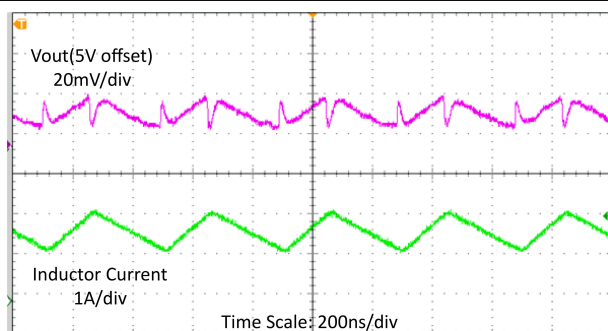
图 7-3. 重负载条件下的开关波形
