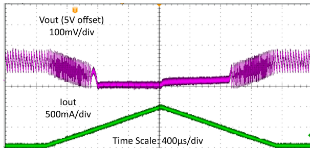
图 7-9. 负载扫描
