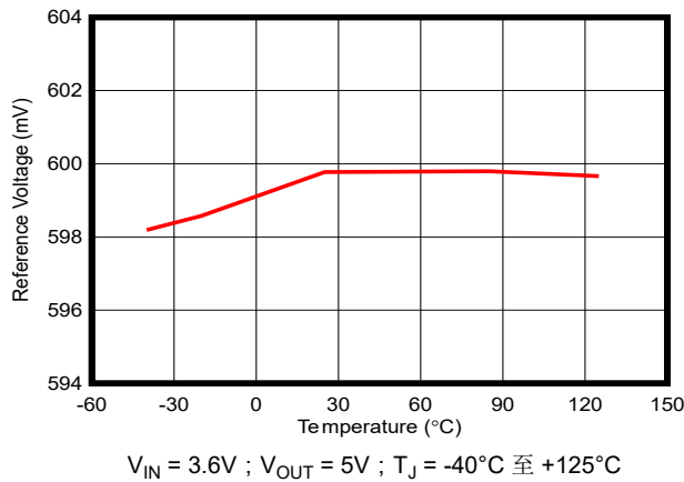
图 5-5. 基准电压与温度间的关系
