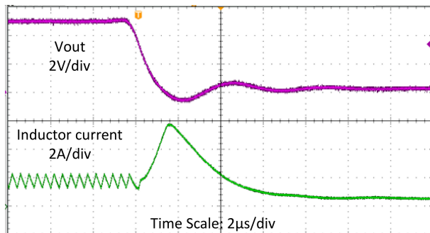
图 7-11. 输出短路保护 (进入)
