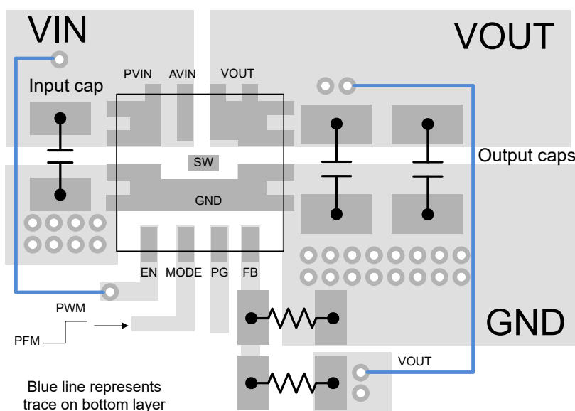
图 7-13. 布局示例
