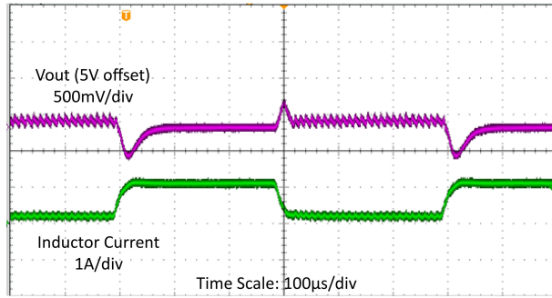
图 7-7. 负载瞬态
