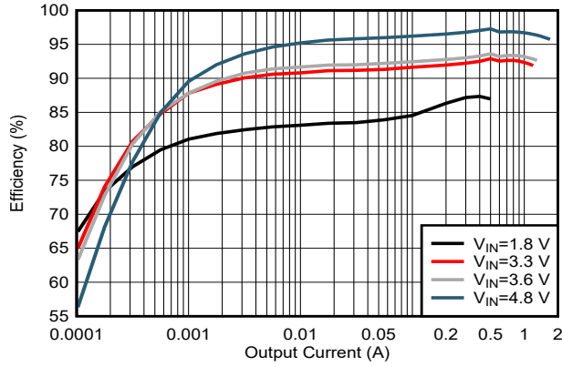
图 5-1. 效率与输出电流间的关系 V_{OUT} = 5V
