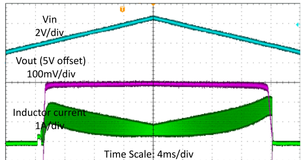
图 7-8. 线路瞬态
