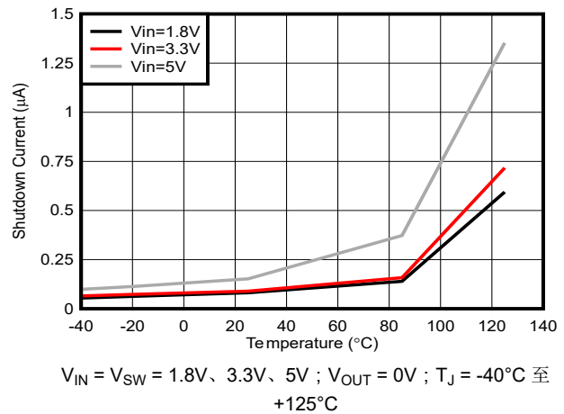
图 5-6. 关断电流与温度间的关系
