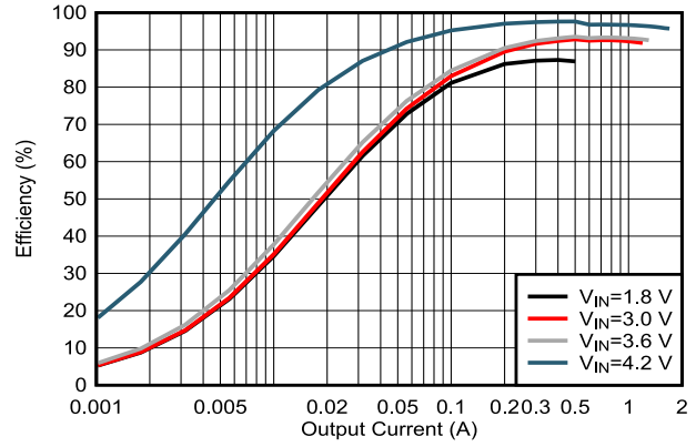
图 5-2. 效率与输出电流间的关系 V_{OUT} = 5V
