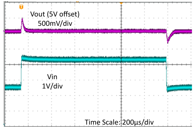
图 7-8. 线路瞬态
