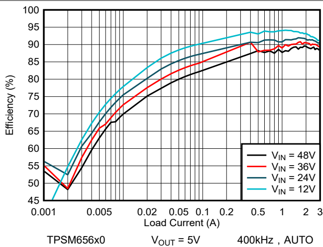
图 8-5. 效率
