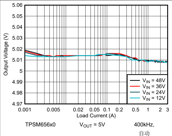
图 8-6. 线性和负载调整率
