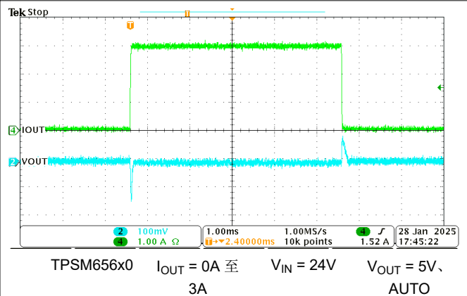
图 8-8. 负载瞬态 (0% 至 100%)
