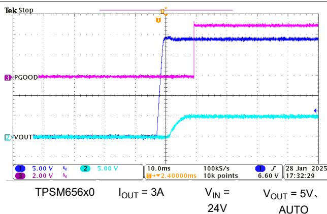
图 8-9. 启动
