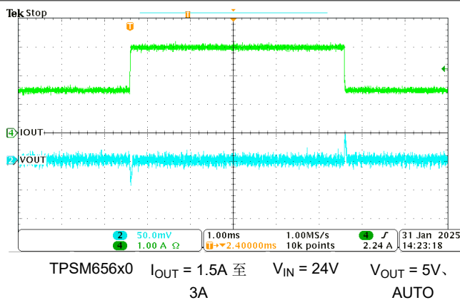
图 8-7. 负载瞬态 (50% 至 100%)
