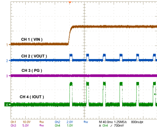
图 8-9. 启动至短路
