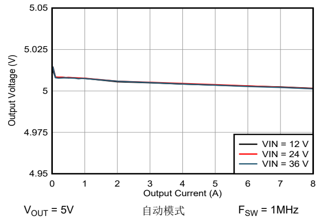
图 8-5. V_{OUT} = 5V 时的负载调节
