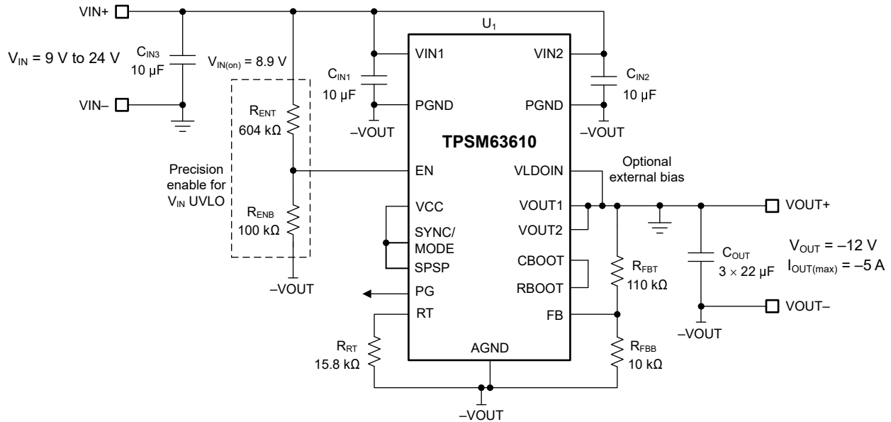
图 8-14. 电路原理图
