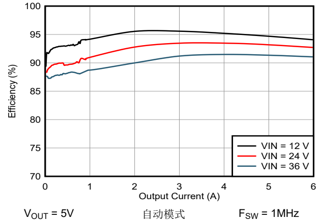
图 9-3. V_{OUT} = 5V 时的效率
