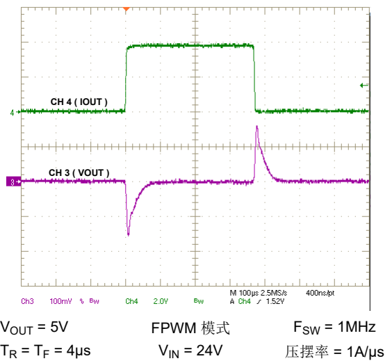
图 9-7. 瞬态负载，在 1A/\mu s 下为 0A 至 4A
