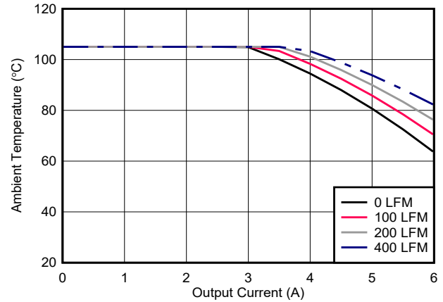
图 7-17. 安全工作区 ( V_{OUT} = 3.3V , F_{SW} = 750\text{kHz} )
