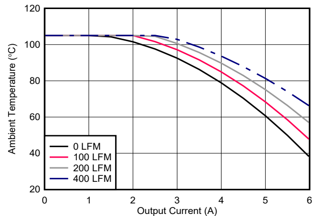
图 7-19. 安全工作区 ( V_{OUT} = 12V , F_{SW} = 2\text{MHz} )
