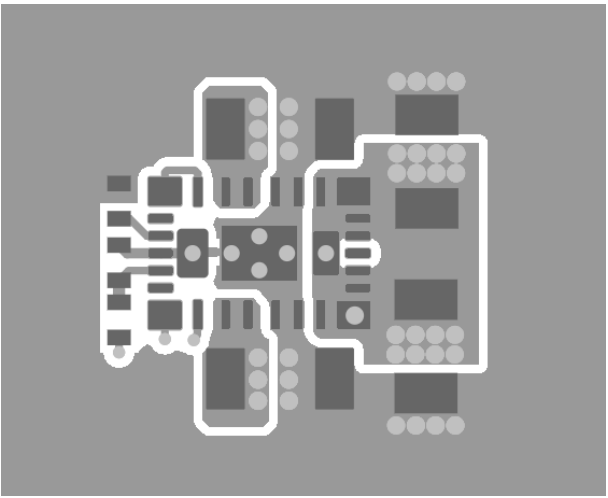
图 11-2. 典型顶层
