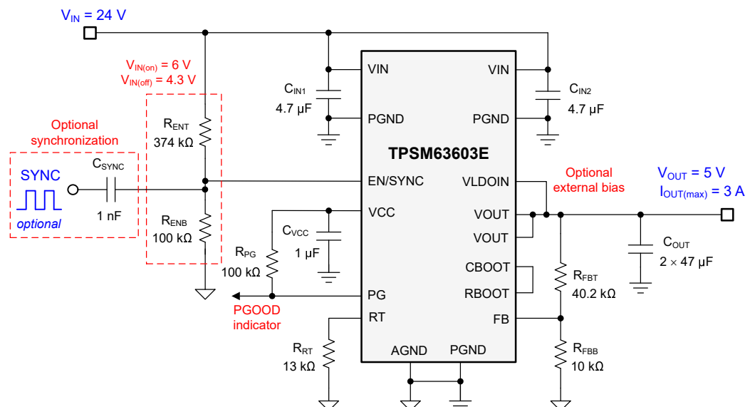
图 9-1. 电路原理图
