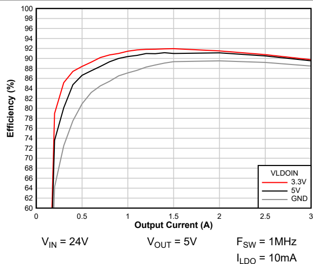
图 7-8. 通过 VLDOIN 实现的效率提升 ( V_{OUT} = 5V )
