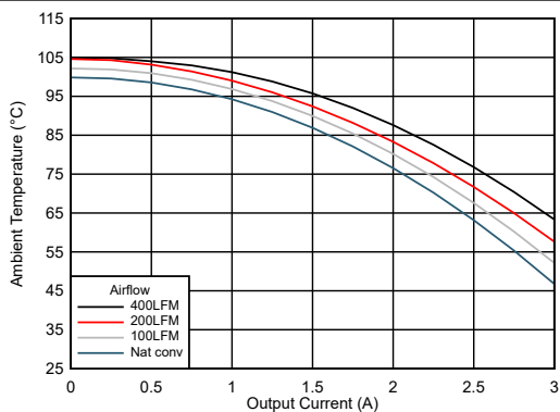
图 6-24. 安全工作区
