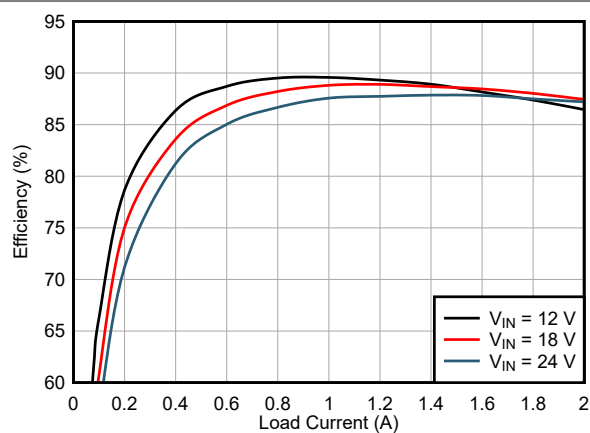
图 8-13. 效率曲线
