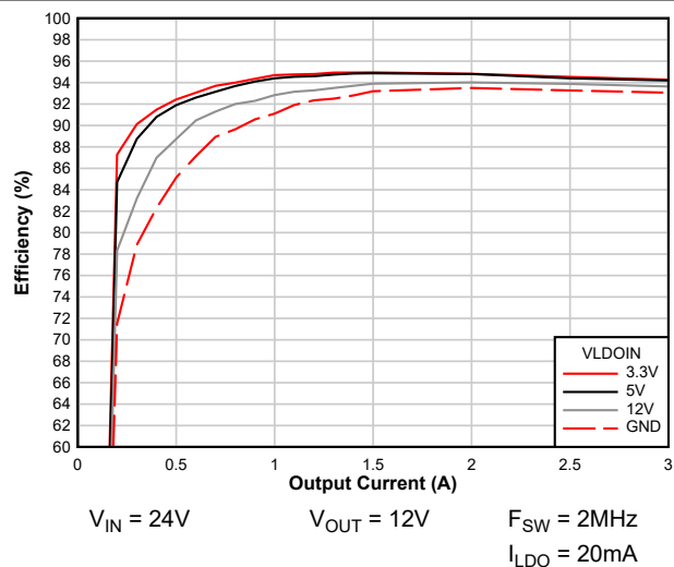
图 7-9. 通过 VLDOIN 实现的效率提升 ( V_{OUT} = 12V )
