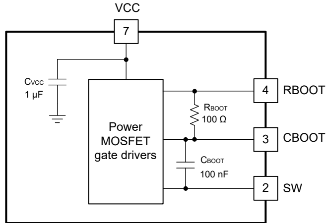
图 7-7. 内部 BOOT 电阻器
