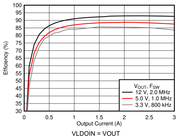
图 6-19. 效率
