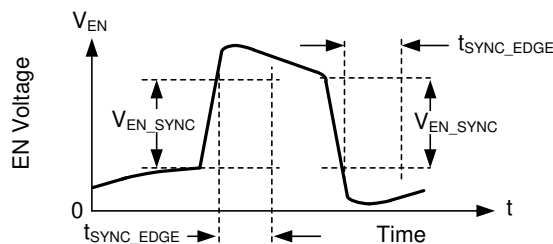
图 7-5. 典型 SYNC 波形
