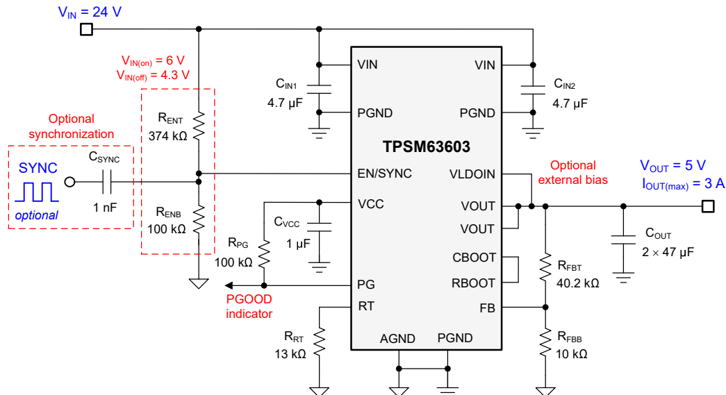
图 8-1. 电路原理图
