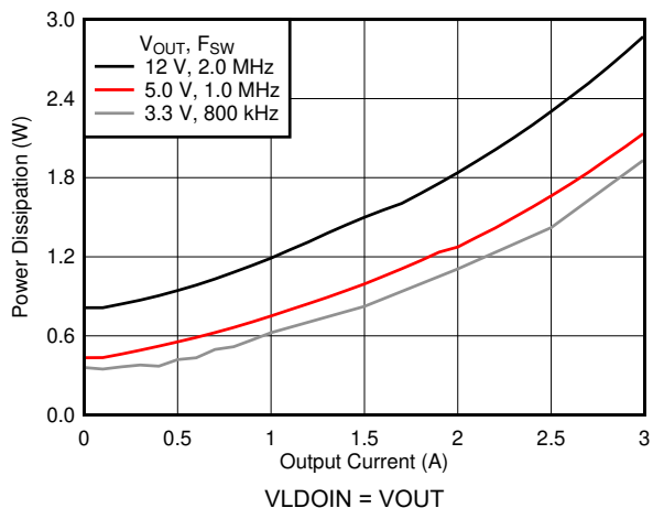
图 6-20. 功率耗散
