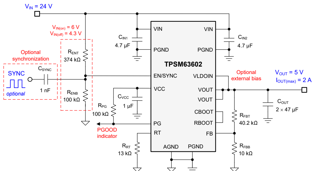
图 9-1. 电路原理图
