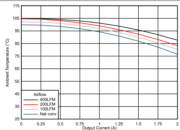
图 7-22. 安全工作区 ( V_{OUT} = 12V )
