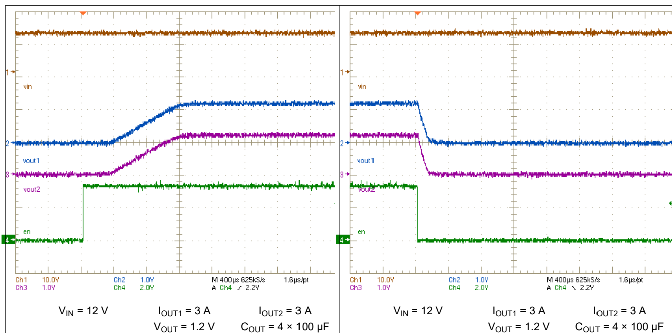
图 8-2. Enable Turn-On with Load
