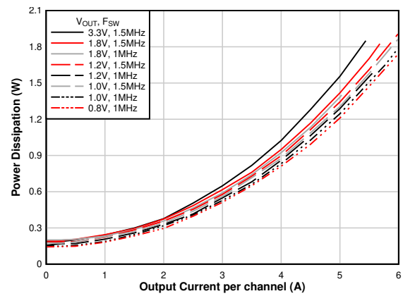
图 6-9. Power Dissipation vs Output Current
