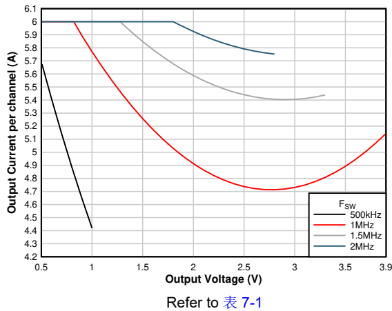
图 6-10. Maximum Output Current
