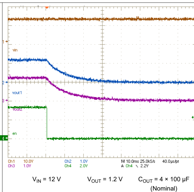
图 8-7. Enable Turn-Off Without Load
