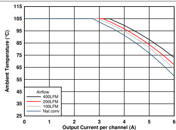
图 6-3. Maximum Output Current
