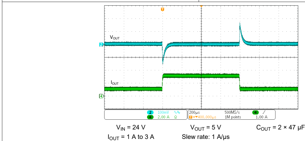
图 8-4. Transient Response
