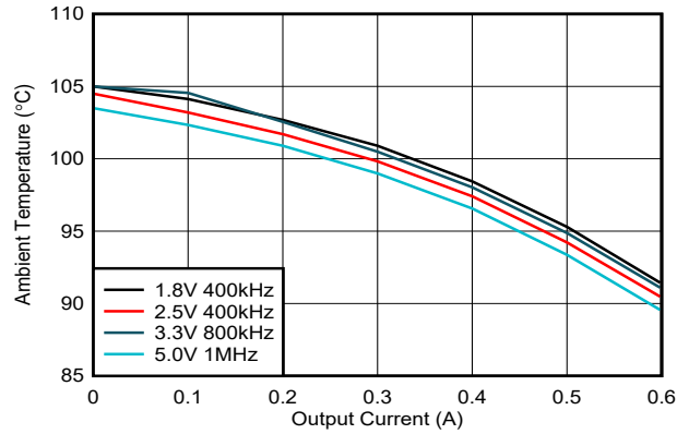
图 8-8. 安全工作区 (标准 EVM 布局和电路板尺寸)
