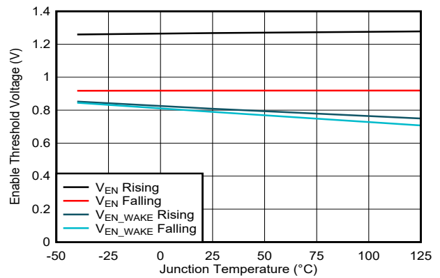
图 8-4. 使能阈值
