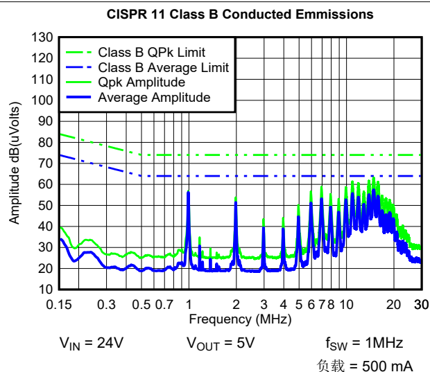
图 10-12. 典型 CISPR 11 B 类传导 EMI 150kHz 至 30MHz, 不带 EMI 滤波器 (标准 EVM 布局和 BOM)
