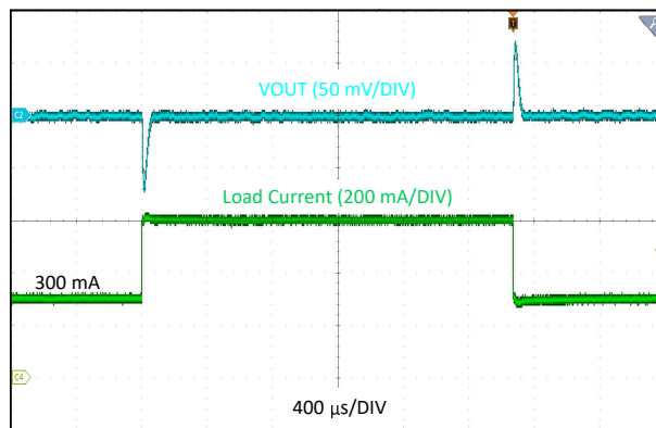
图 10-6. 瞬态负载，在 1A/\mu s 下为 0.3 A 至 0.6 A
