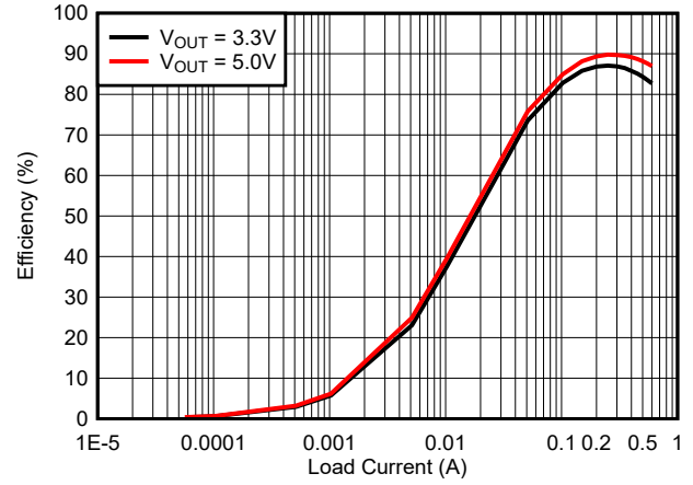
图 8-7. FPWM 模式下的效率
