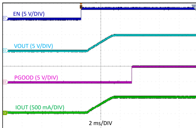
图 9-4. V_{IN} = 24V 、 V_{OUT} = 5V 、 I_{OUT} = 0.5A 时的使能启动
