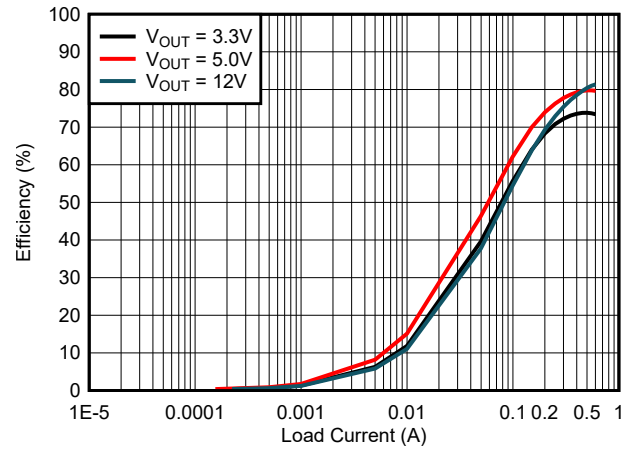
图 8-13. FPWM 模式下的效率
