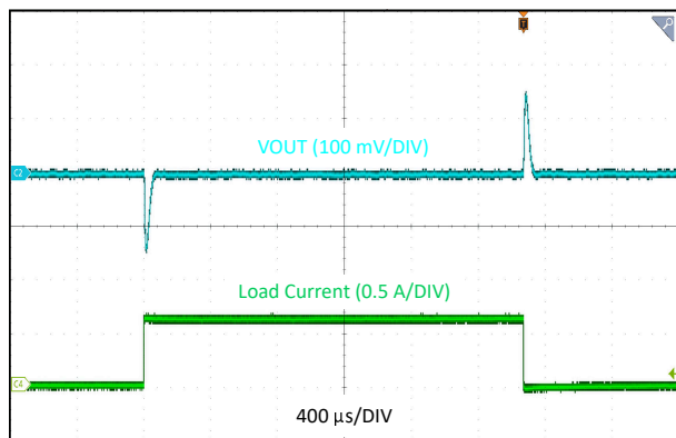
图 10-5. 瞬态负载，在 1A/\mu s 下为 0A 至 0.6 A
