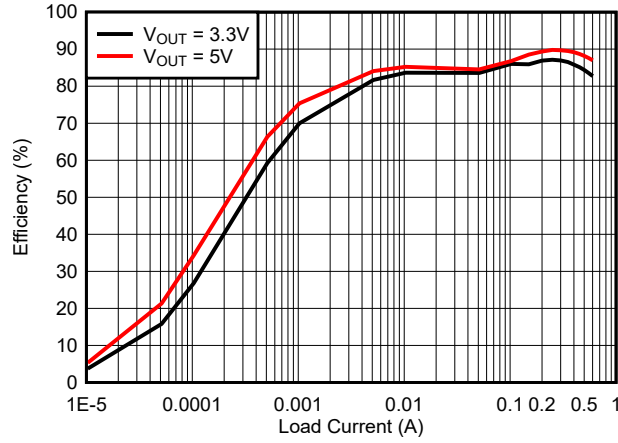
图 8-6. 自动模式下的效率
