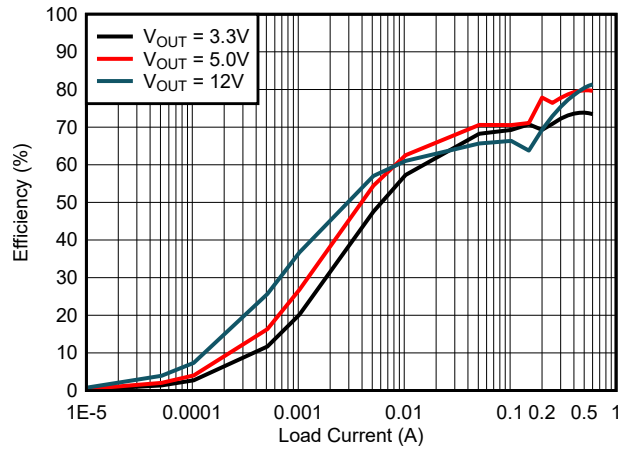
图 8-12. 自动模式下的效率
