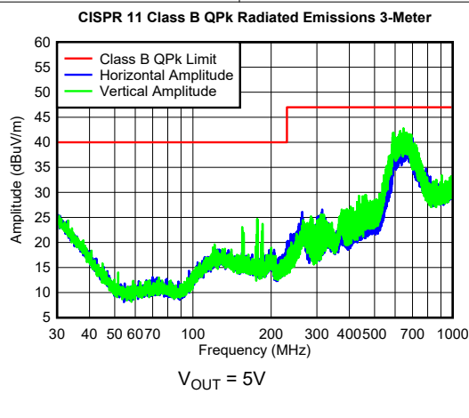
图 10-13. 典型 CISPR 11 B 类辐射 EMI 30kHz 至 1000MHz (标准 EVM 布局和 BOM, 去除了输入滤波器)
