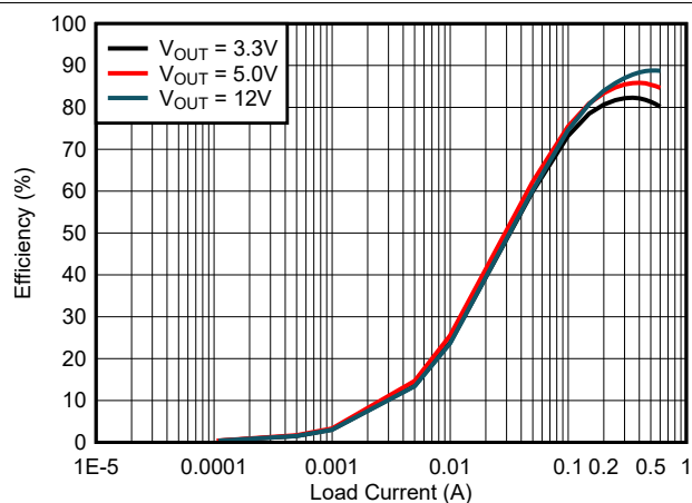
图 8-10. FPWM 模式下的效率
