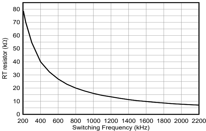
图 9-9. RT 值与频率间的关系
