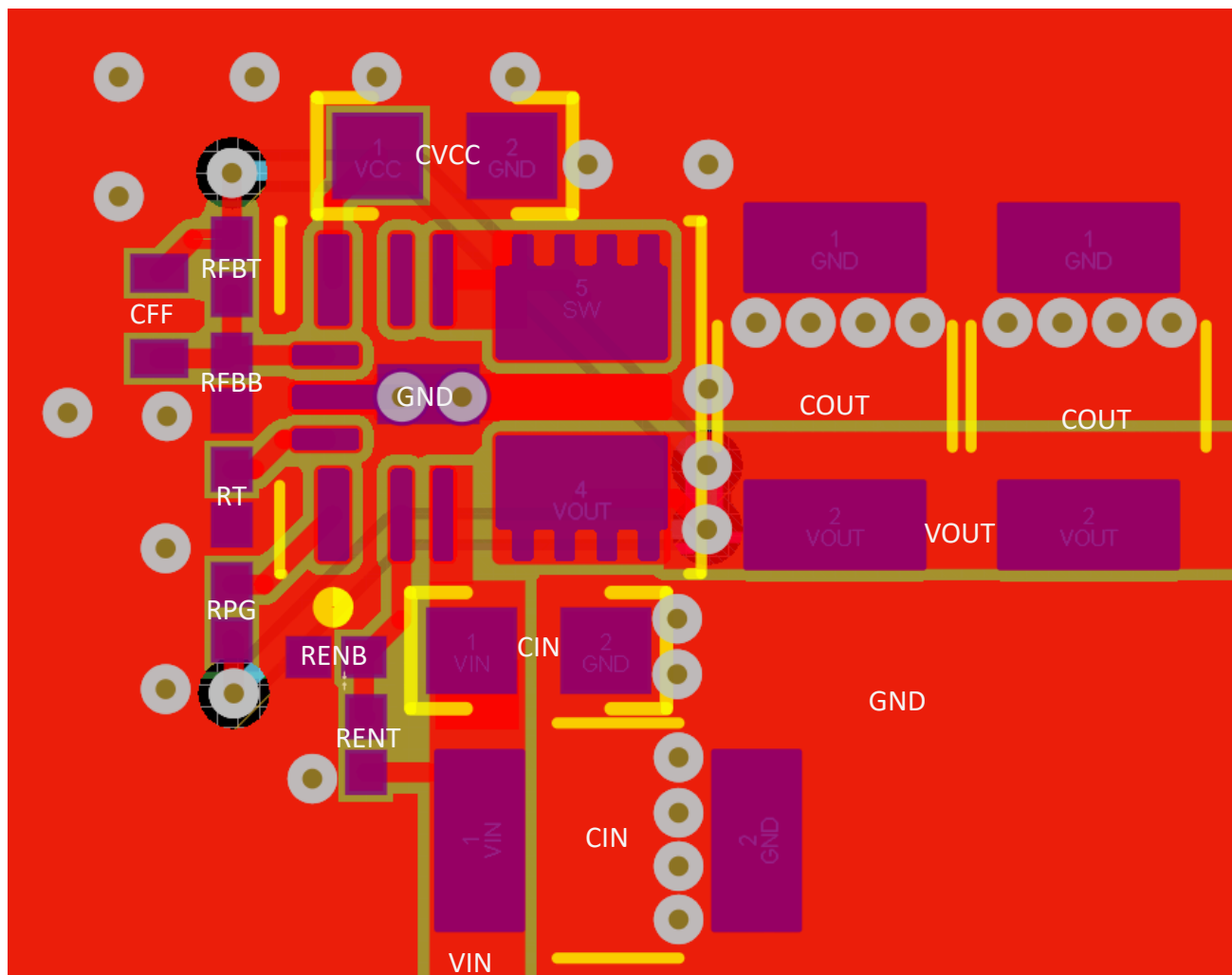
图 10-15. 布局示例
