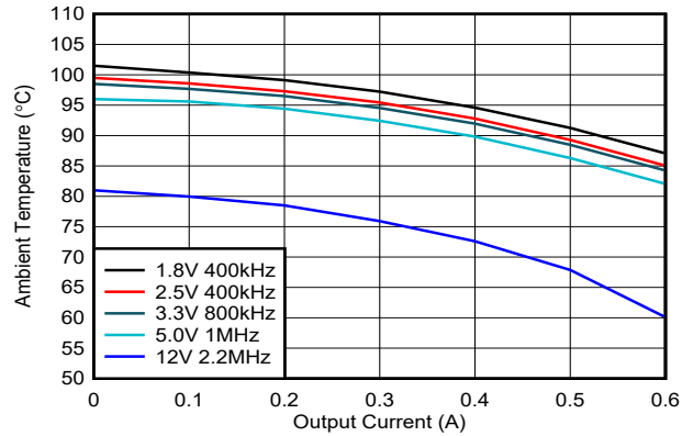
图 8-14. 安全工作区 (标准 EVM 布局和电路板尺寸)
