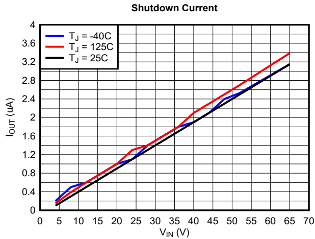
图 8-1. 关断电源电流
