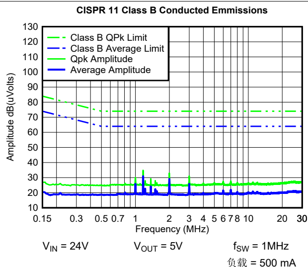
图 10-11. 典型 CISPR 11 B 类传导 EMI 150kHz 至 30MHz, 带 EMI 滤波器 (标准 EVM 布局和 BOM)
