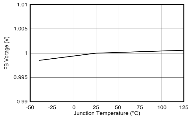
图 8-2. 反馈电压
