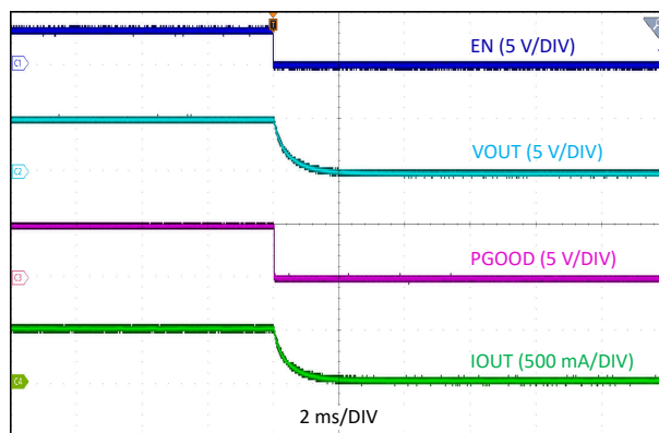
图 10-4. 关断波形
