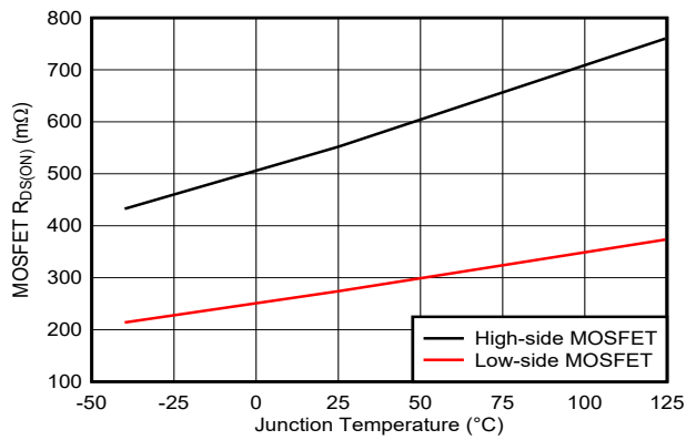
图 8-3. 高侧与低侧 MOSFET R_{DS(on)}
