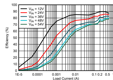
效率与输出电流间的关系 V_{\text{OUT}} = 5\text{V} , F_{\text{sw}} = 1\text{MHz}
