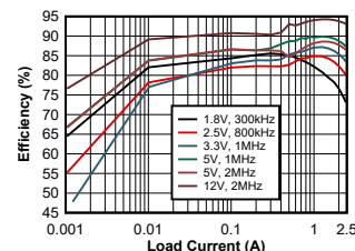
效率与输出电流间的关系 V_{IN} = 24V
