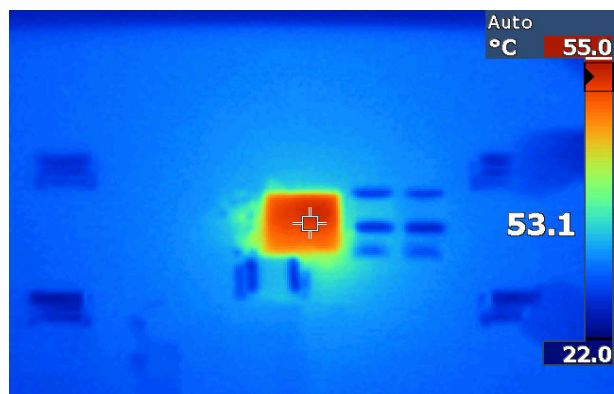
图 8-16. EVM 热性能
