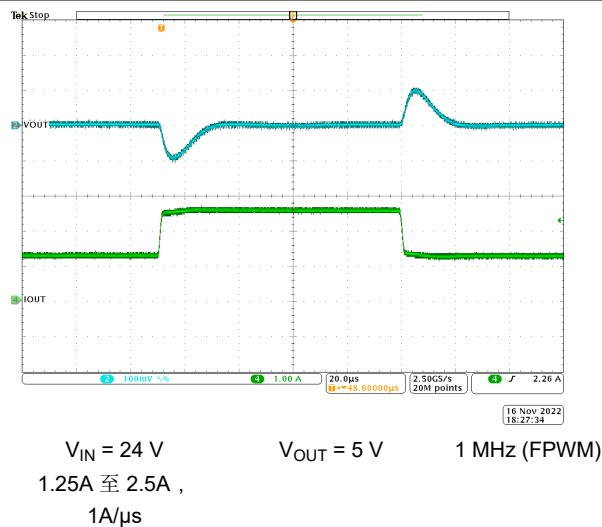
图 8-13. 负载瞬态
