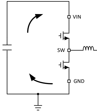
图 8-22. 具有快速边沿的电流环路
