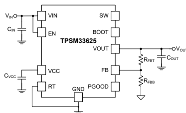
典型电路原理图
