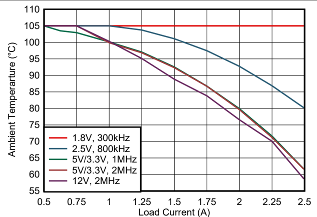
图 8-8. 24VIN : 最高环境温度与负载电流间的关系 (对 TPSM33625EVM 的分析)
