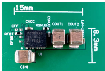
EVM 布局典型设计尺寸 – 15mm × 8.3mm
