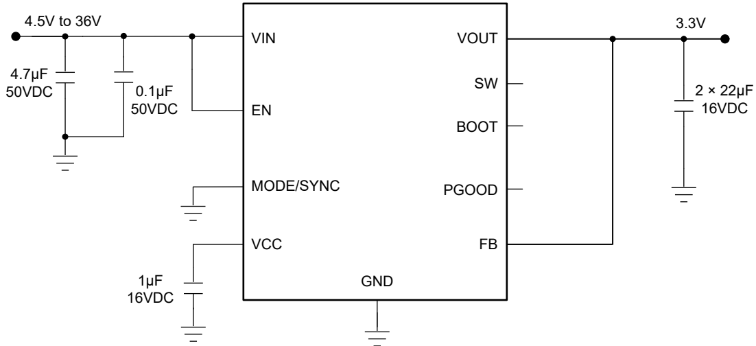
图 8-2. 3.3V VOUT 设计示例
