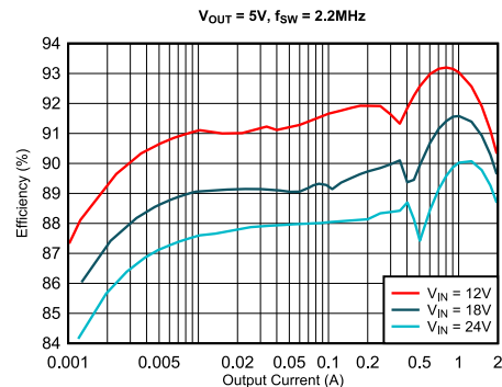
效率与输出电流之间的关系
