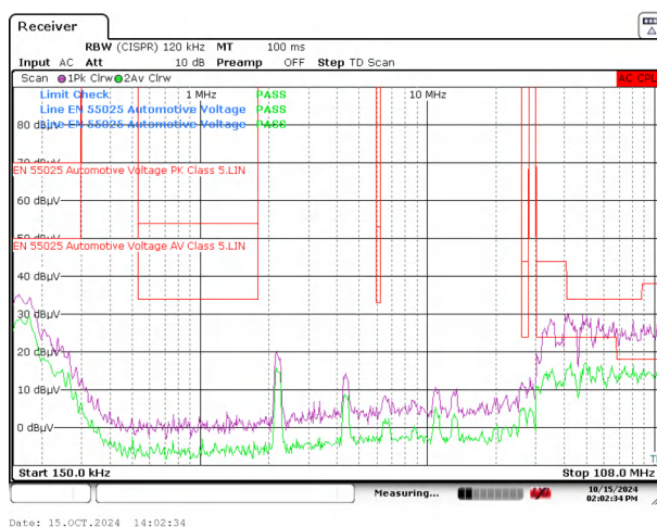
图 8-6. CISPR 25, CE 扫描 150kHz - 108MHz, (紫色峰值、绿色 AVG), 12VIN, 3.3VOUT, 2.2MHz, 2A 负载电流
