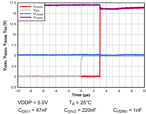
图 6-3. t LH_VDRV
