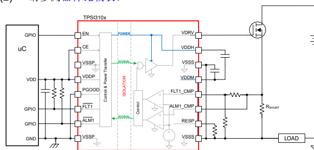
TPSI3100-Q1 简化原理图
