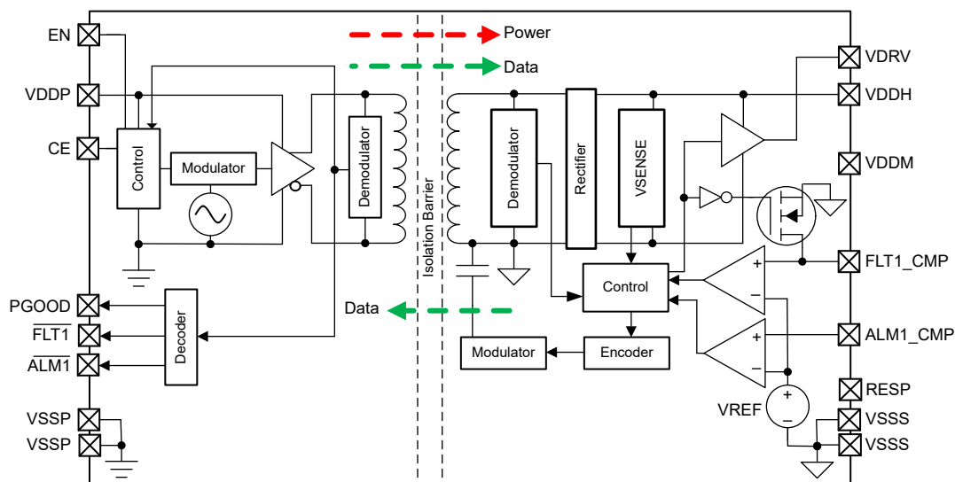
图 8-4. TPSI3133-Q1
