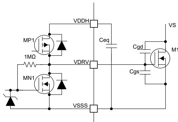
图 8-9. 禁止电路
