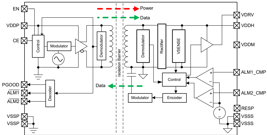
图 8-3. TPSI312x-Q1
