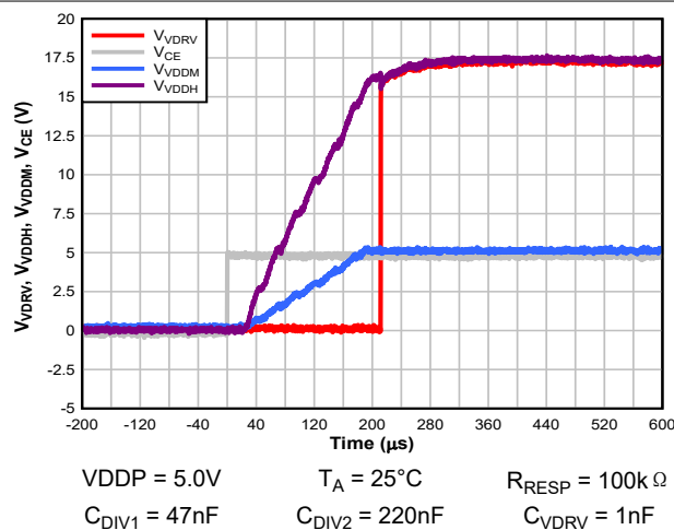
图 6-7. t LH_VDRV_CE
