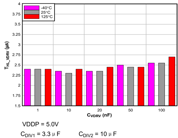
图 6-6. t HL_VDRV 与 C VDRV
