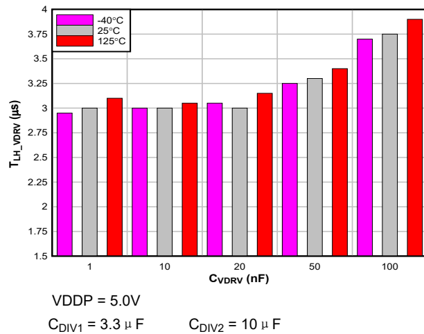
图 6-5. t LH_VDRV 与 C VDRV
