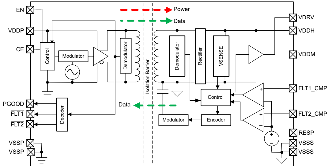
图 8-2. TPSI311x、TPSI311xL
