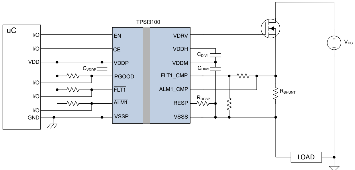
图 9-1. TPSI3100 通过故障和警报指示器提供过流保护
