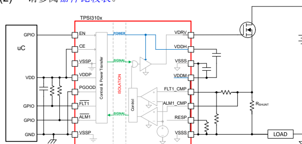
TPSI3100 简化原理图
