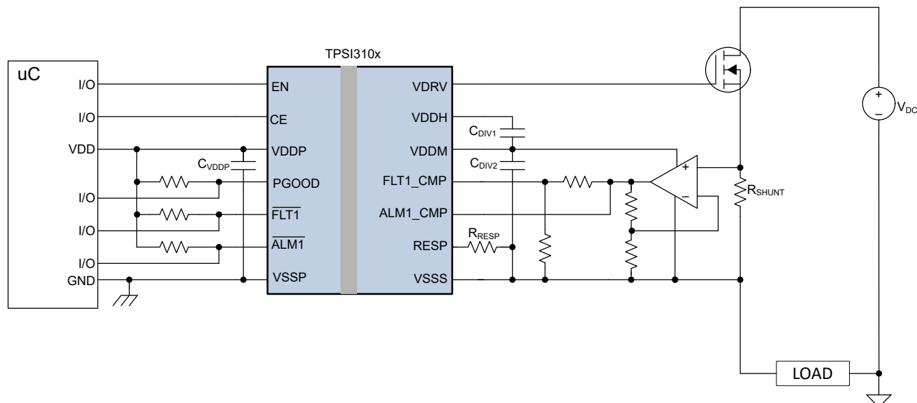
图 9-2. TPSI310x 通过电流检测放大器、故障和警报指示器提供过流保护
