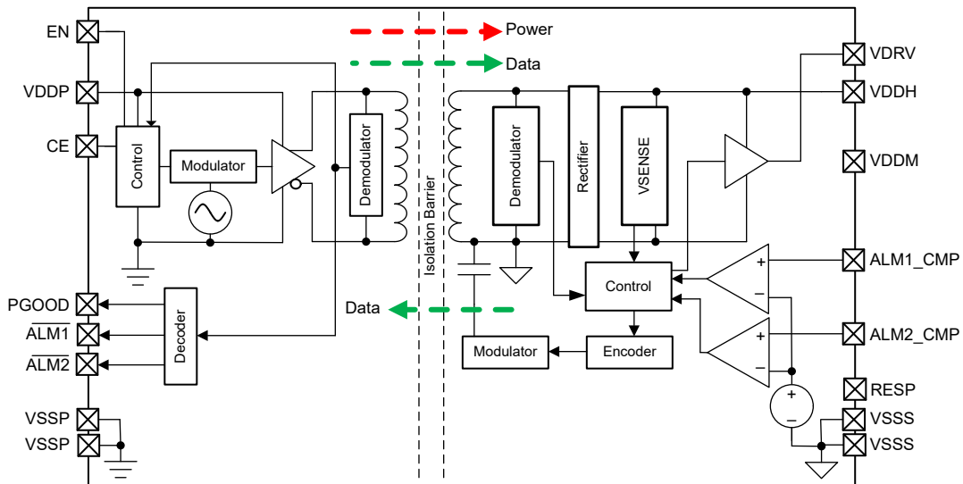
图 8-3. TPSI312x
