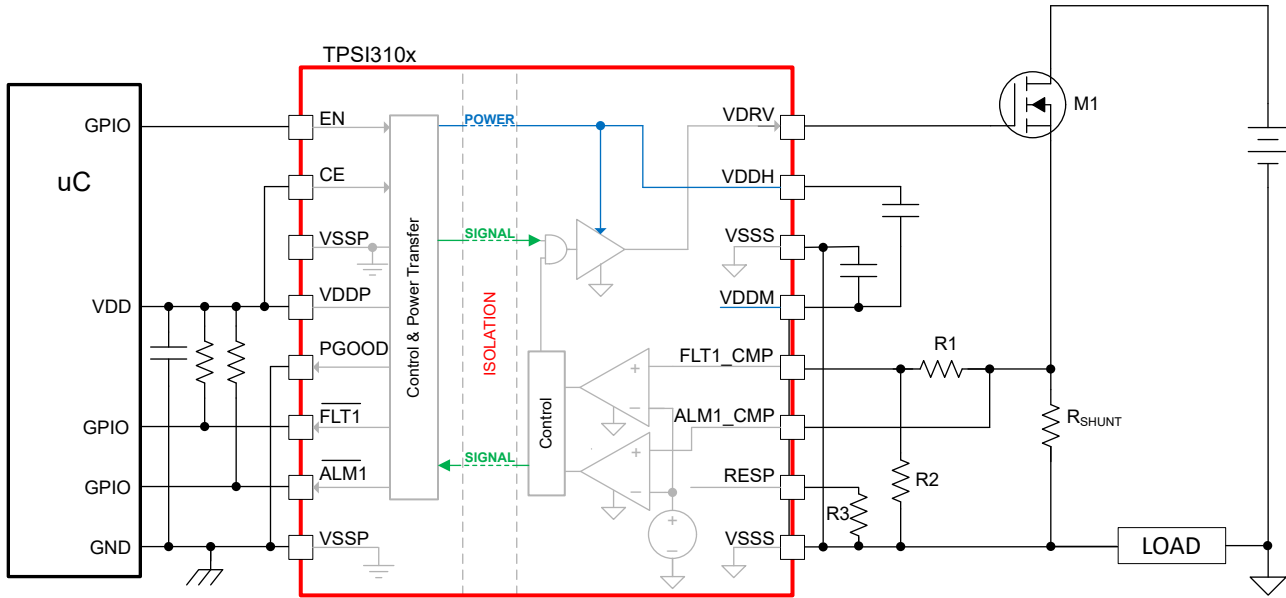
图 9-6. 典型过流保护应用
