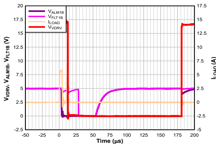
图 9-8. 过流保护和 VDRV 自动恢复
