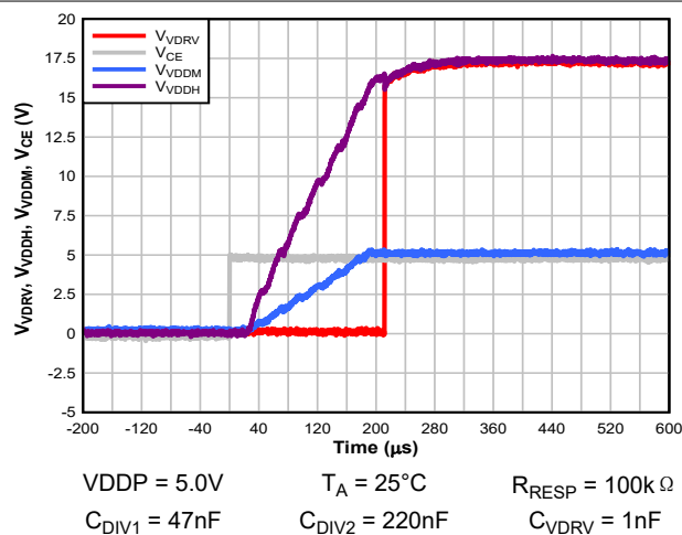
图 6-7. t LH_VDRV_CE
