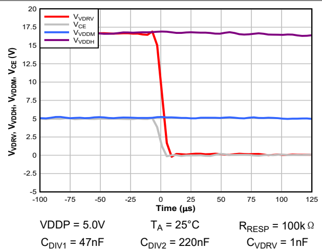
图 6-8. t HL_VDRV_CE (放大图)
