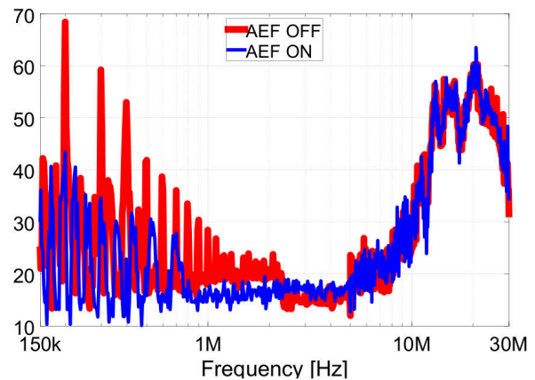
EMI 降噪结果
