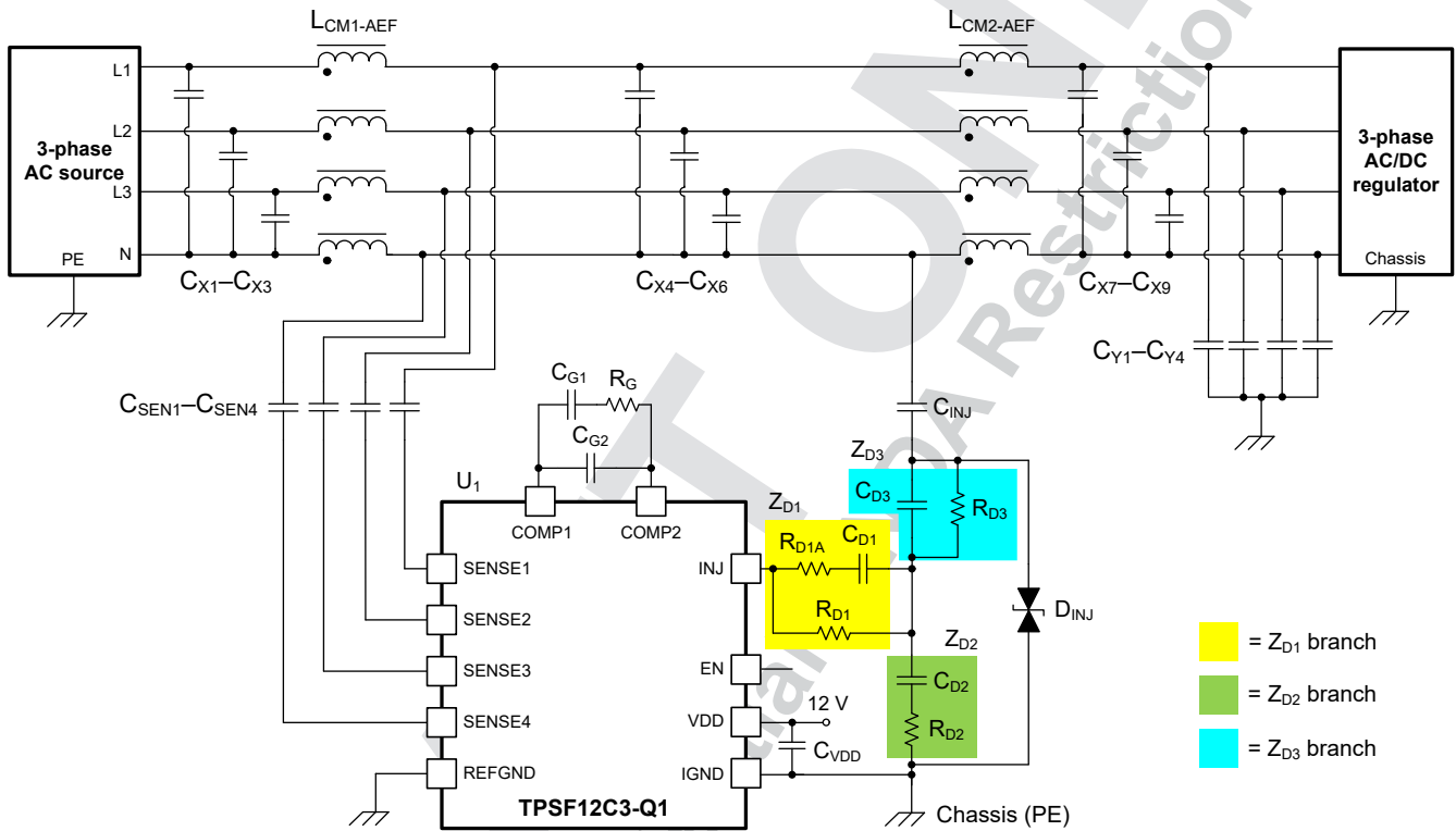
图 9-3. 注入网络
