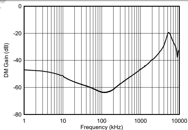
图 7-6. 输入滤波器响应 - 差分模式
