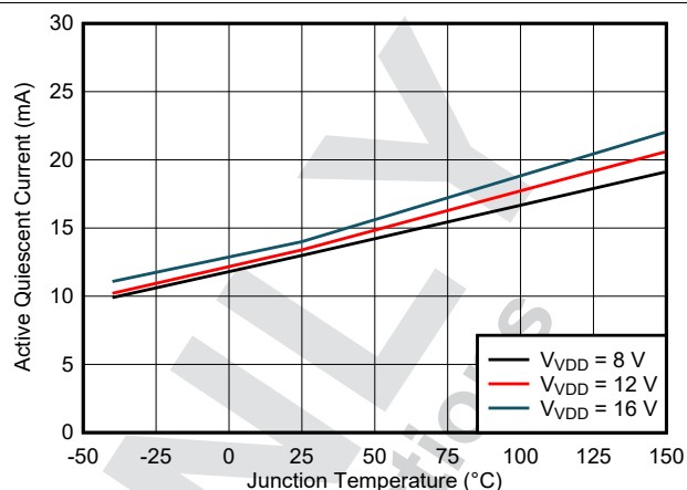
图 7-2. 静态电源电流与温度间的关系
