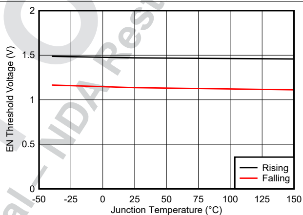
图 7-4. EN 阈值与温度间的关系
