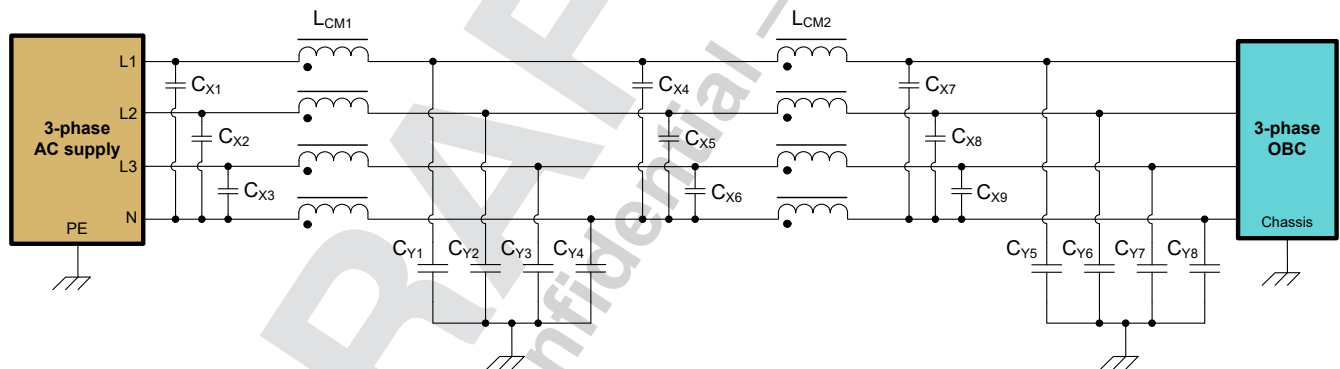
图 9-1. 采用传统两级无源 EMI 滤波器的三相 OBC 的电路原理图
