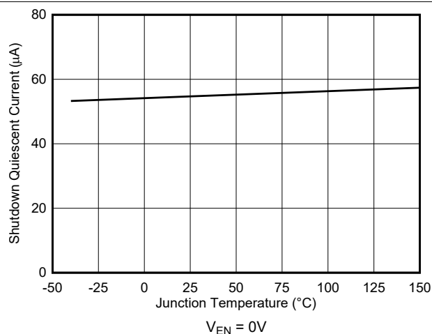
图 7-1. 关断电源电流与温度间的关系
