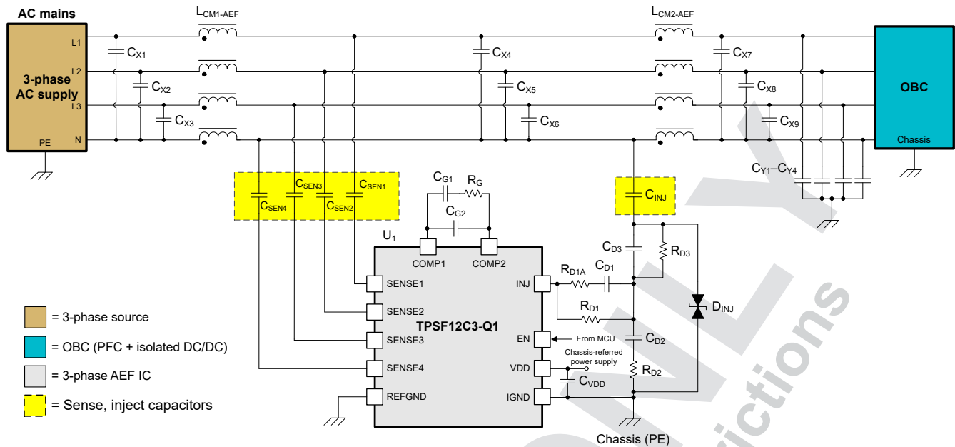
图 9-2. 连接了 AEF 电路的三相 OBC 的电路原理图
