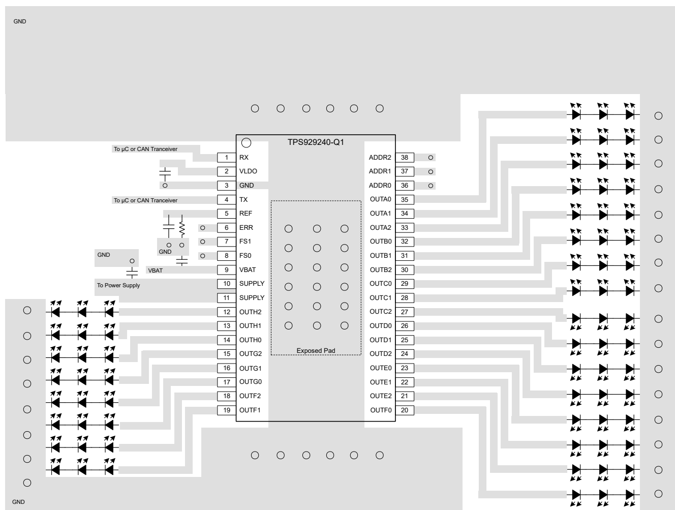
图 7-5. TPS929240-Q1 Layout
