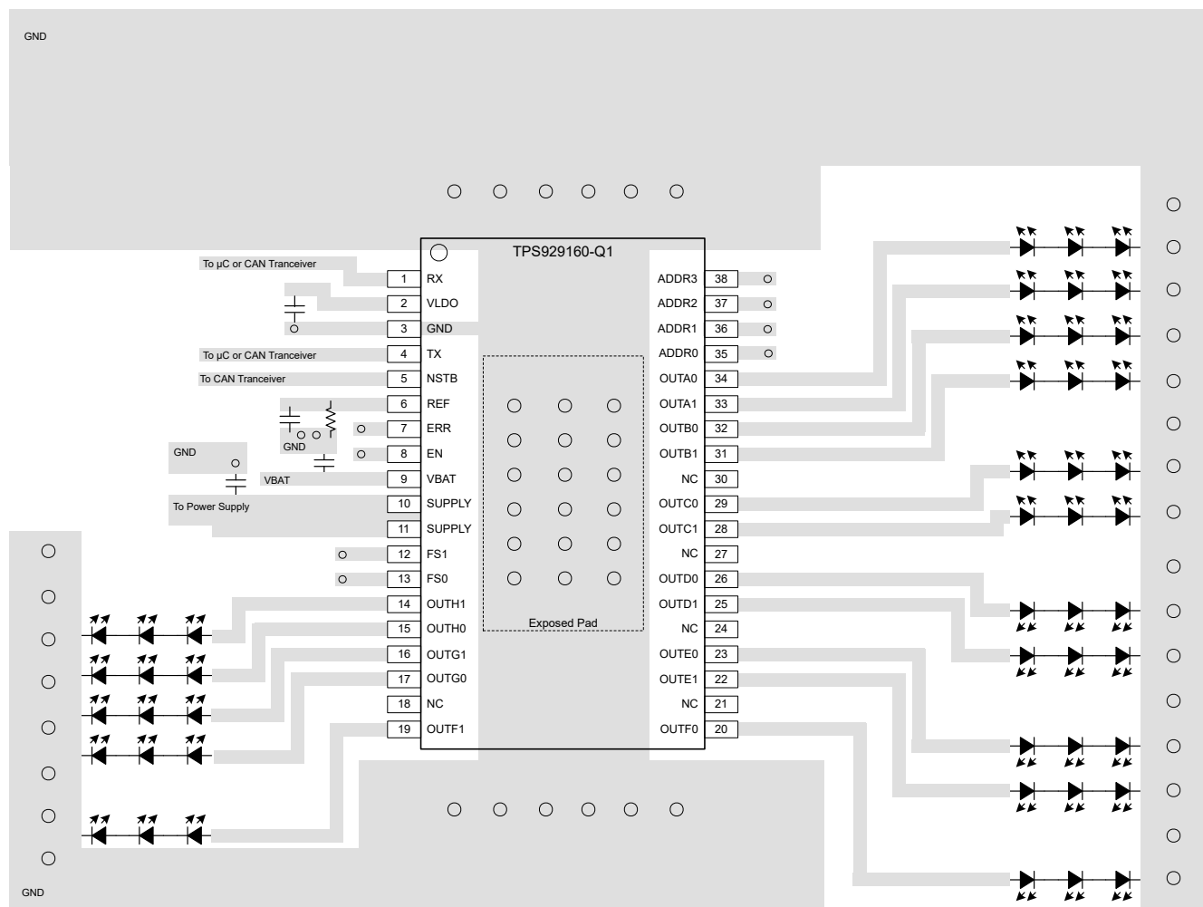
图 7-5. TPS929160-Q1 Layout
