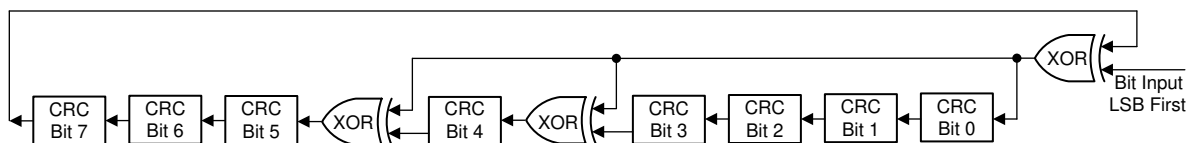
图 6-9. CRC Algorithm Diagram
