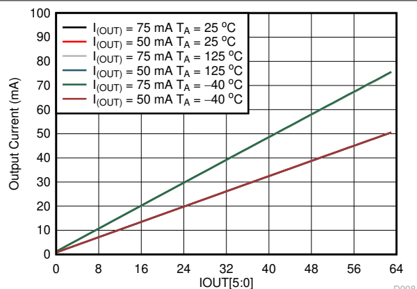
图 6-8. Output DC Current vs IOUT[5:0]
