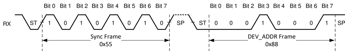
图 7-13. Synchronization Byte
