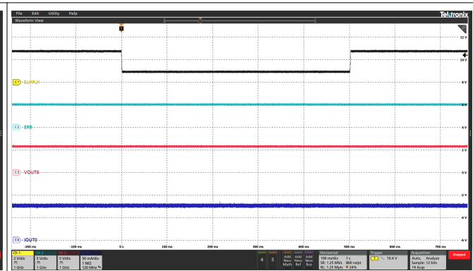
图 6-14. Transient Undervoltage
