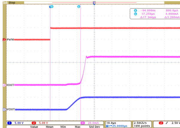
图 24. Output Current With PWM Input
