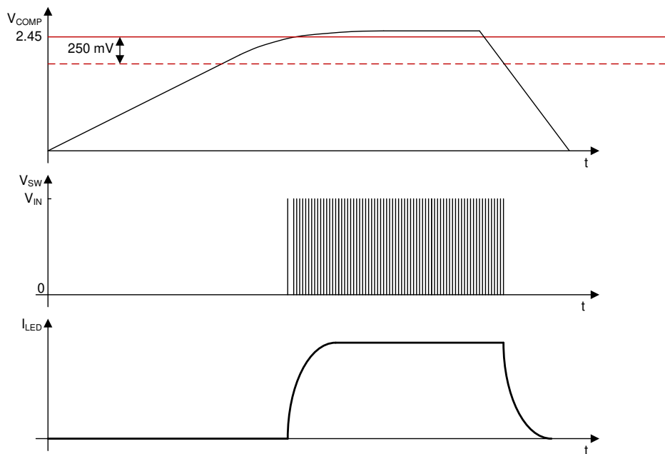
图 7-3. Soft-Start Sequence
