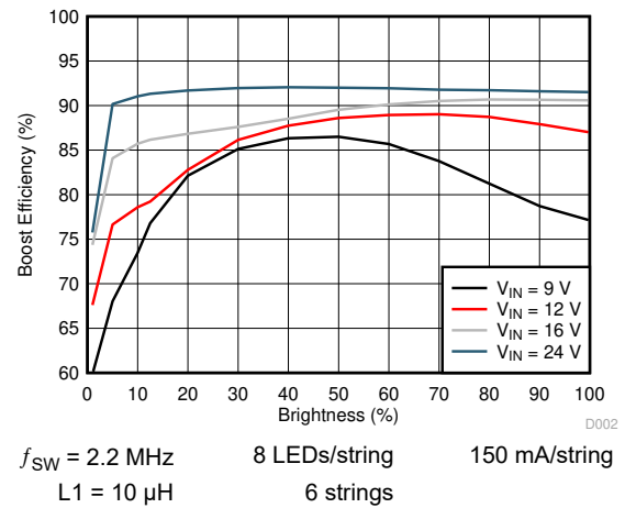
图 6-3. Boost Efficiency
