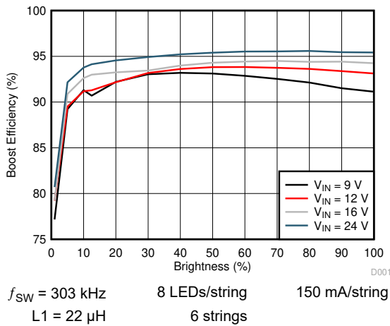
图 6-2. Boost Efficiency
