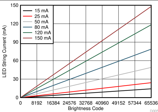
图 6-6. Current Linearity
