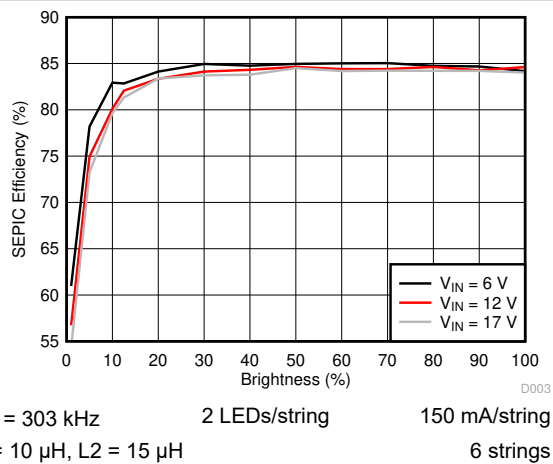
图 6-4. SEPIC Efficiency
