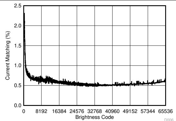
图 6-7. Current Matching
