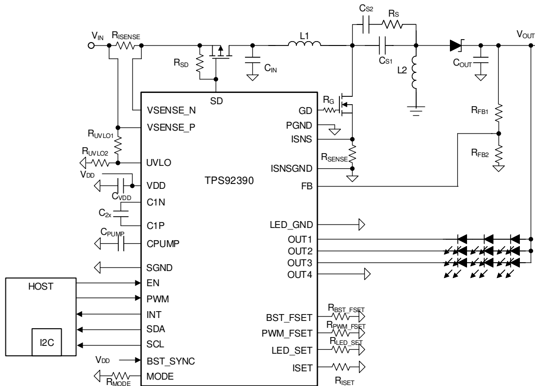
图 8-6. SEPIC 模式与三个 LED 串联
