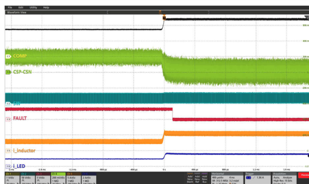
黑色：COMP，浅蓝色：SW，红色：FAULT，橙色：电感器电流，深蓝色：LED 电流，绿色：CSP-CSN
