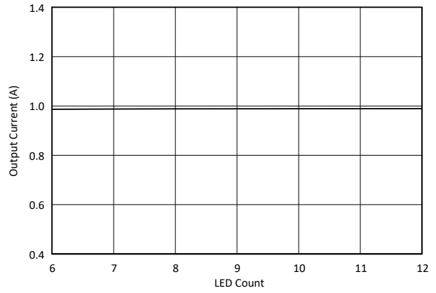
图 6-2. 输出电流与 LED 计数间的关系
