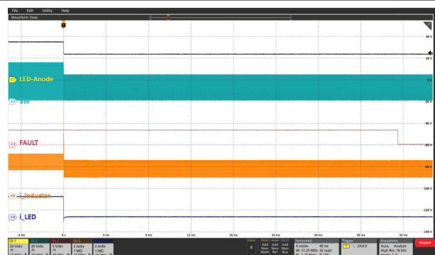
黑色： PWM_{PWM} ，浅蓝色：SW，红色：FAULT，橙色：电感器电流，深蓝色：LED 电流
