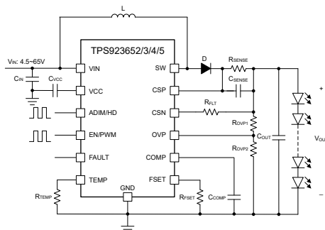
简化原理图
