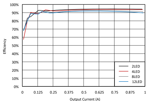
图 6-12. 13V 输入电压、1A 输出电流下的效率
