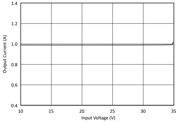
图 6-1. 输出电流与输入电压间的关系
