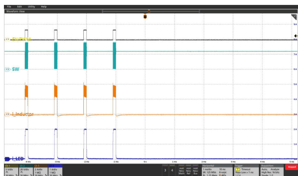
图 8-20. 在 PWM PWM = 100%、1kHz 时关断
